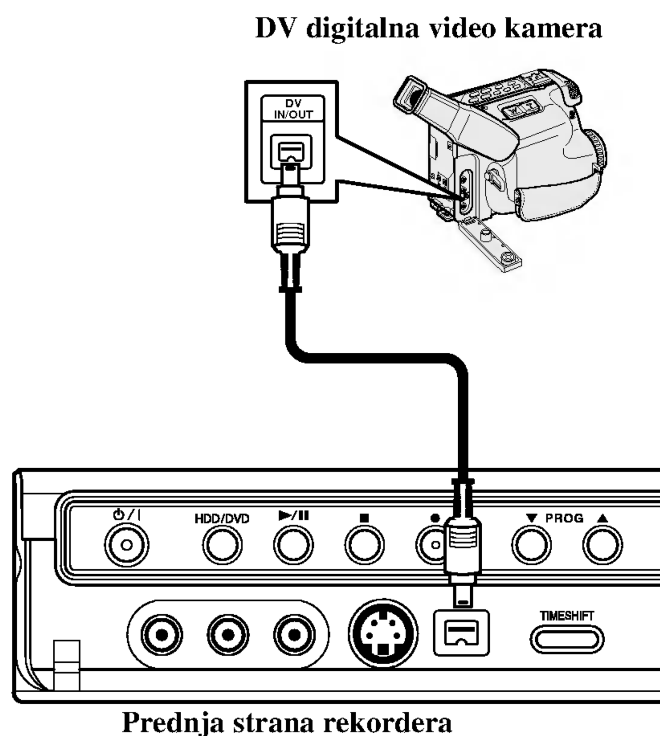
Prednja strana rekordera
