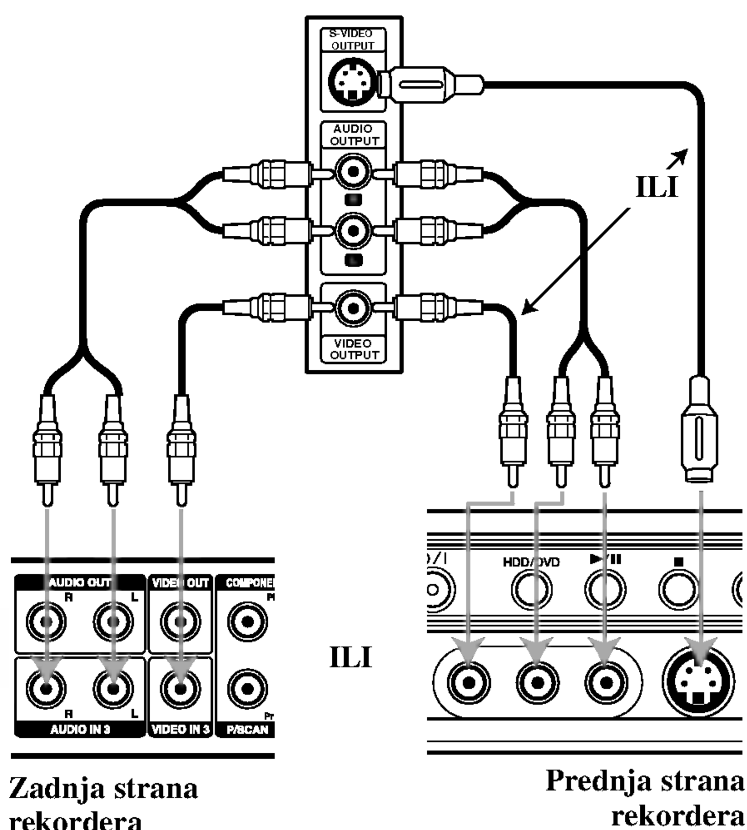
Ploča s konektorom dodatne komponente (VCR, video kamera, i sl.)
