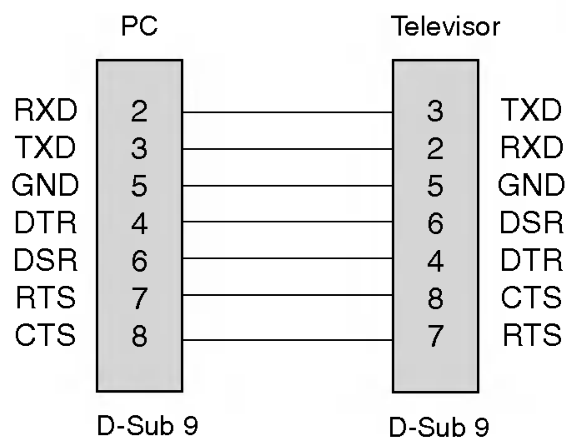
Configuraciones de 7 cables (cable estándar RS-232C)
