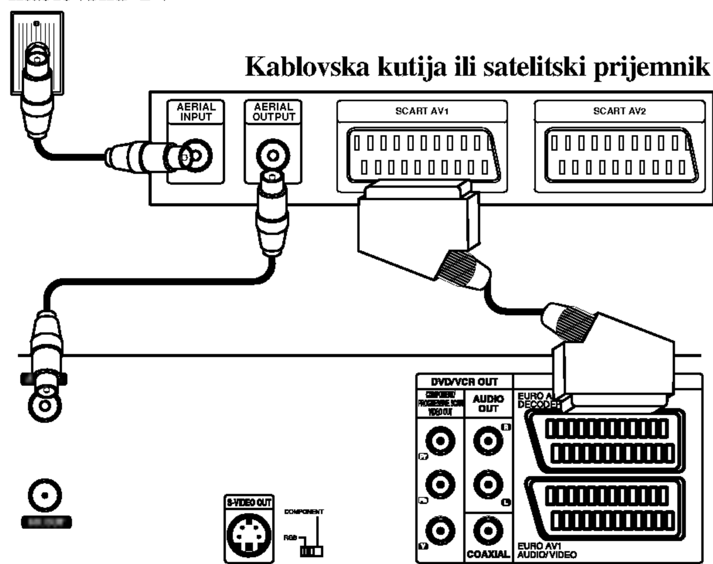
Zidna utičnica za Antenu/ kablovsku TV
