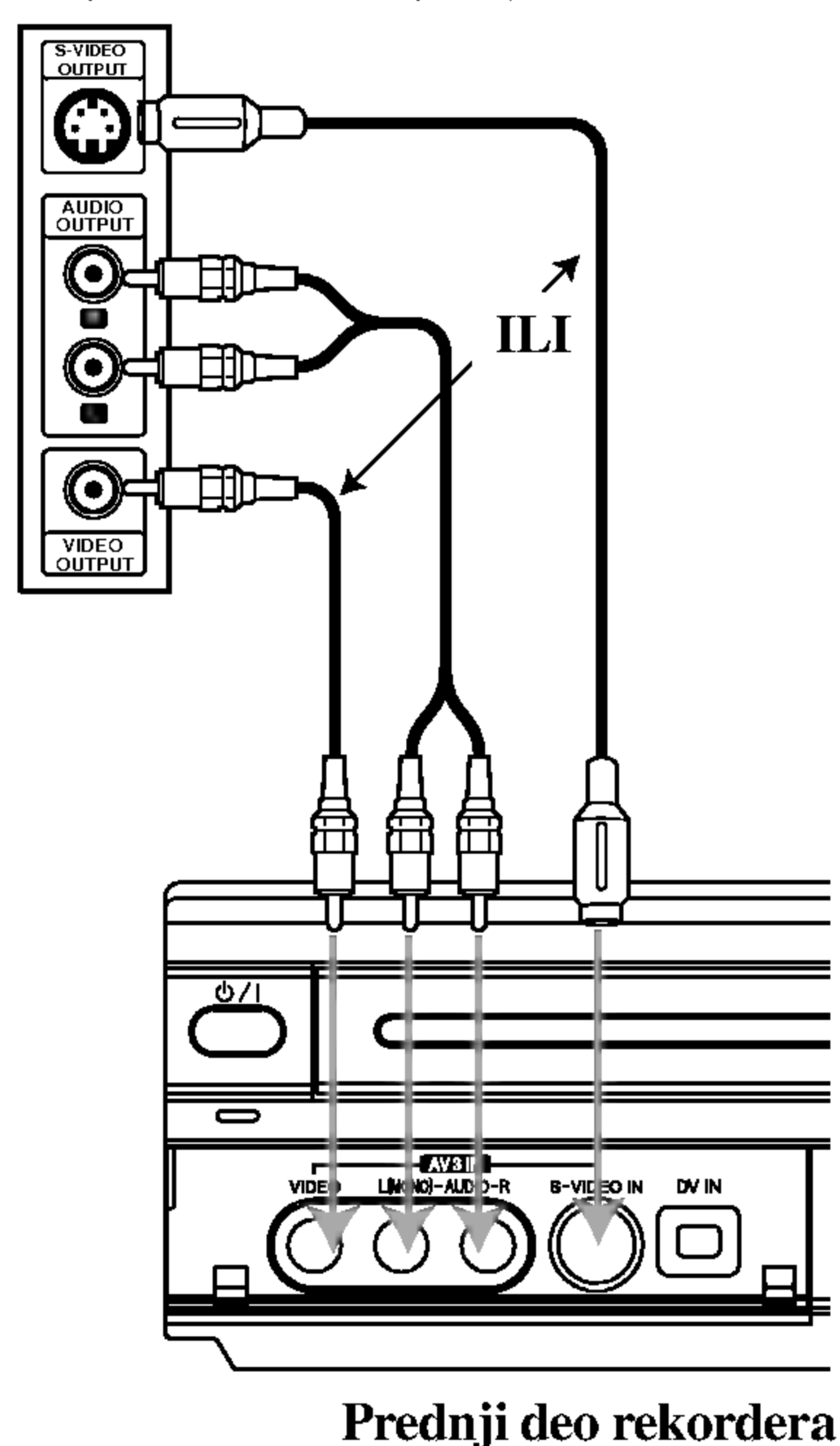
Panel sa utičnicama dodatnih komponenti (video rekorder, video kamera, itd.)
