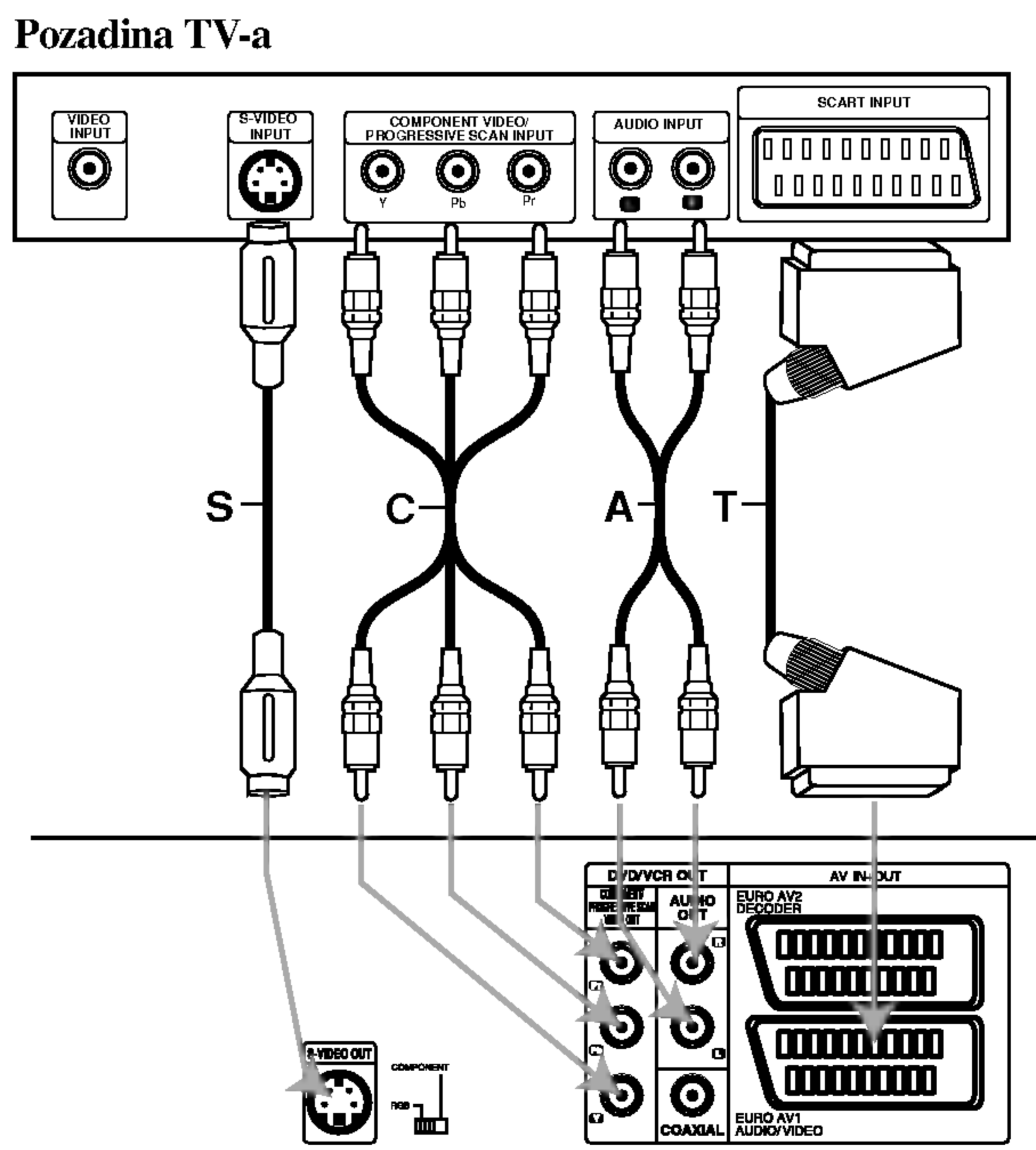
Pozadina rekordera
