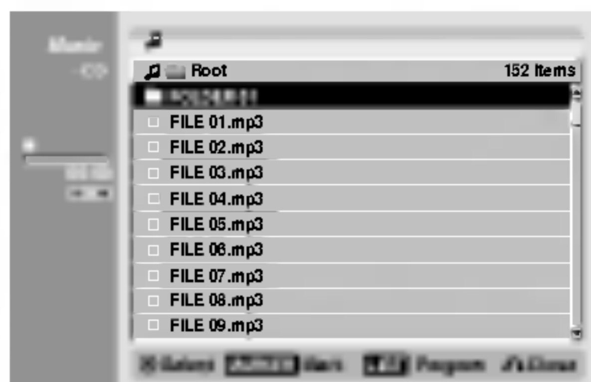
Meni MP3/WMA
