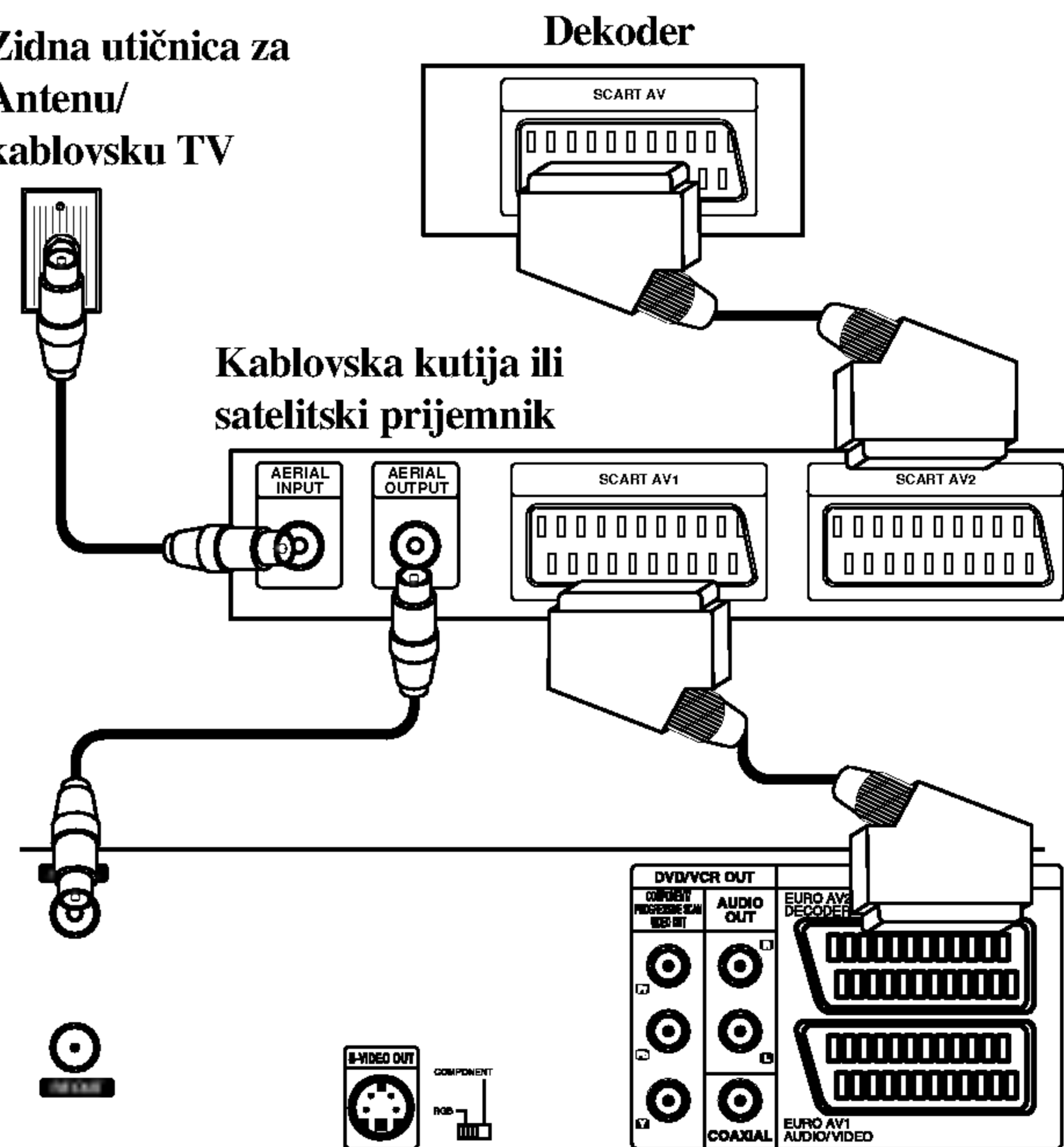
Pozadina rekordera
