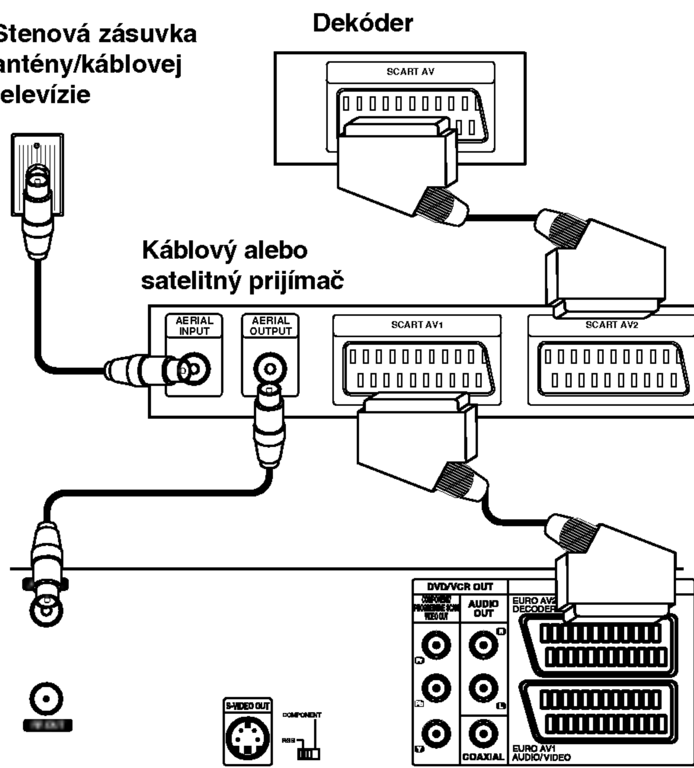
Zadný panel rekordéra
