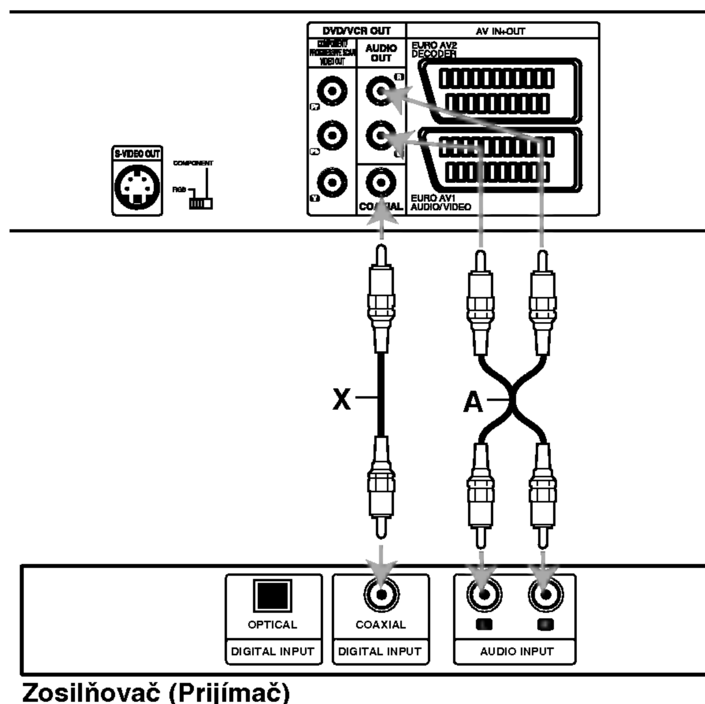
Zadný panel rekordéra
