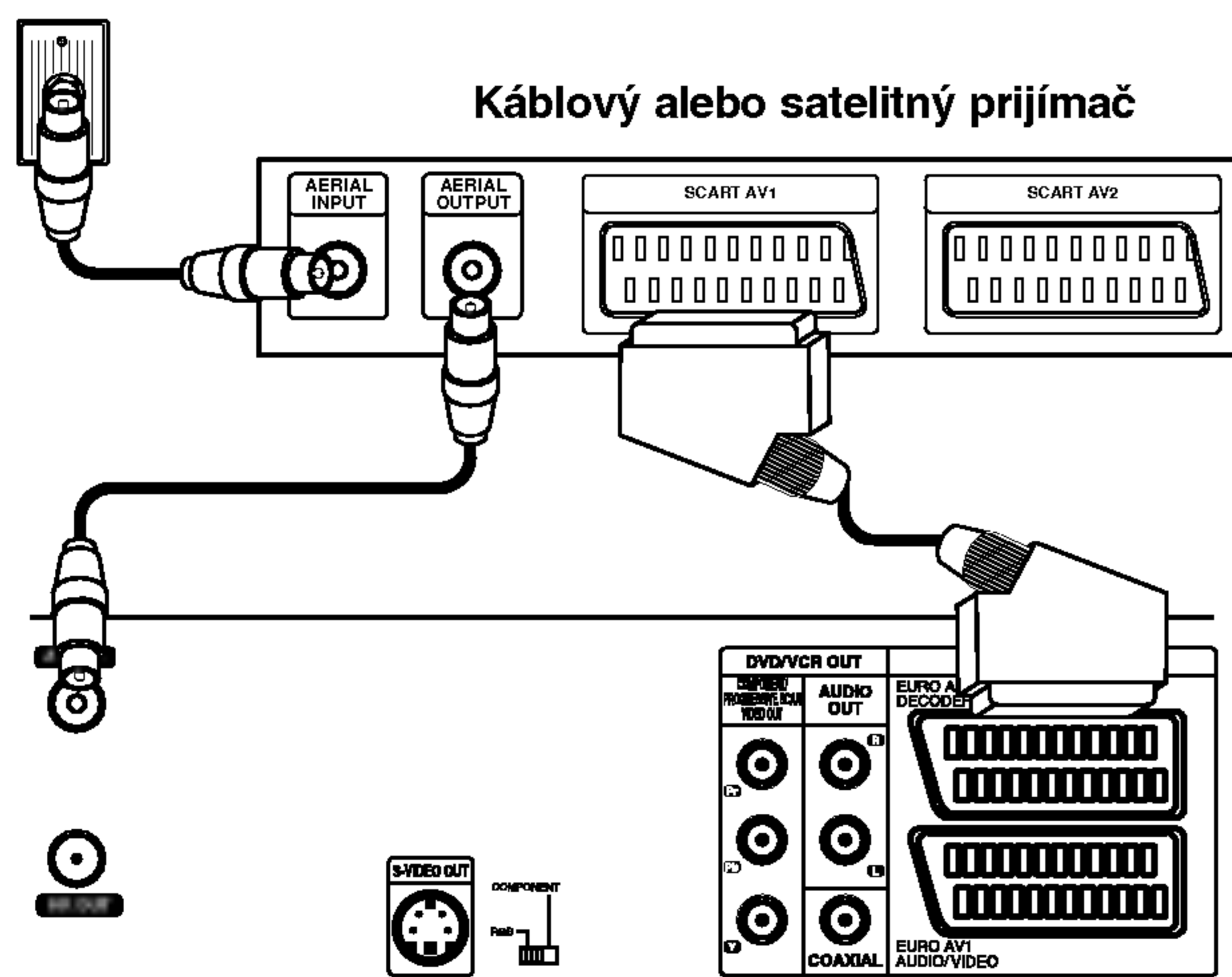
Zadný panel rekordéra
