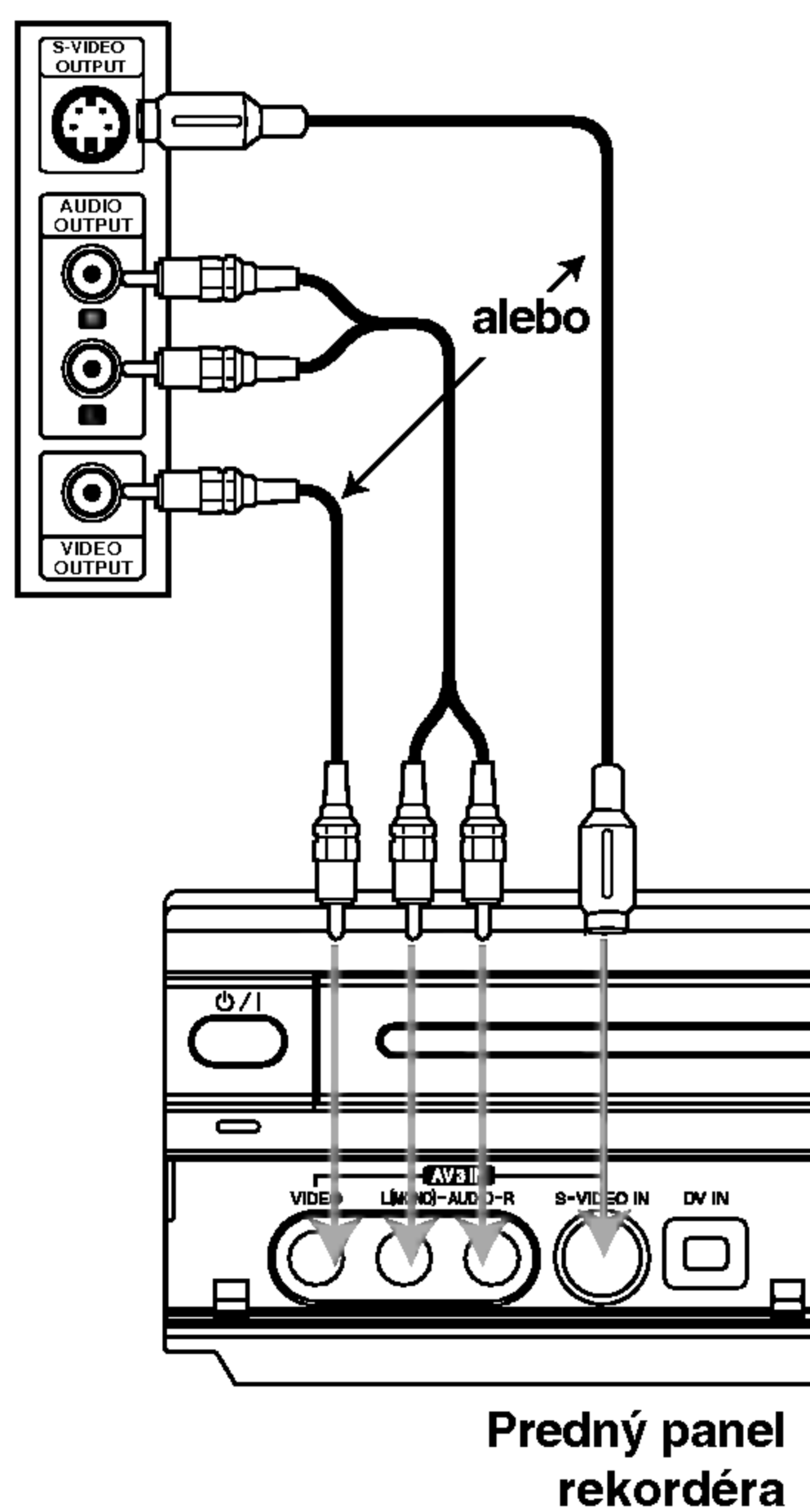
Panel koncoviek prídavného zariadenia (video rekordér, kamera atď.)
