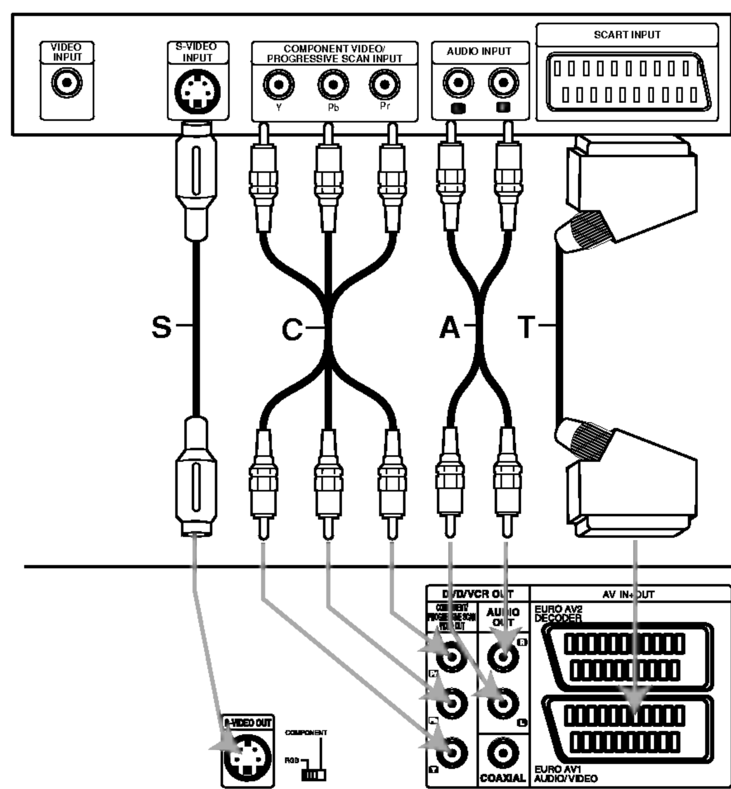
Zadný panel rekordéra
