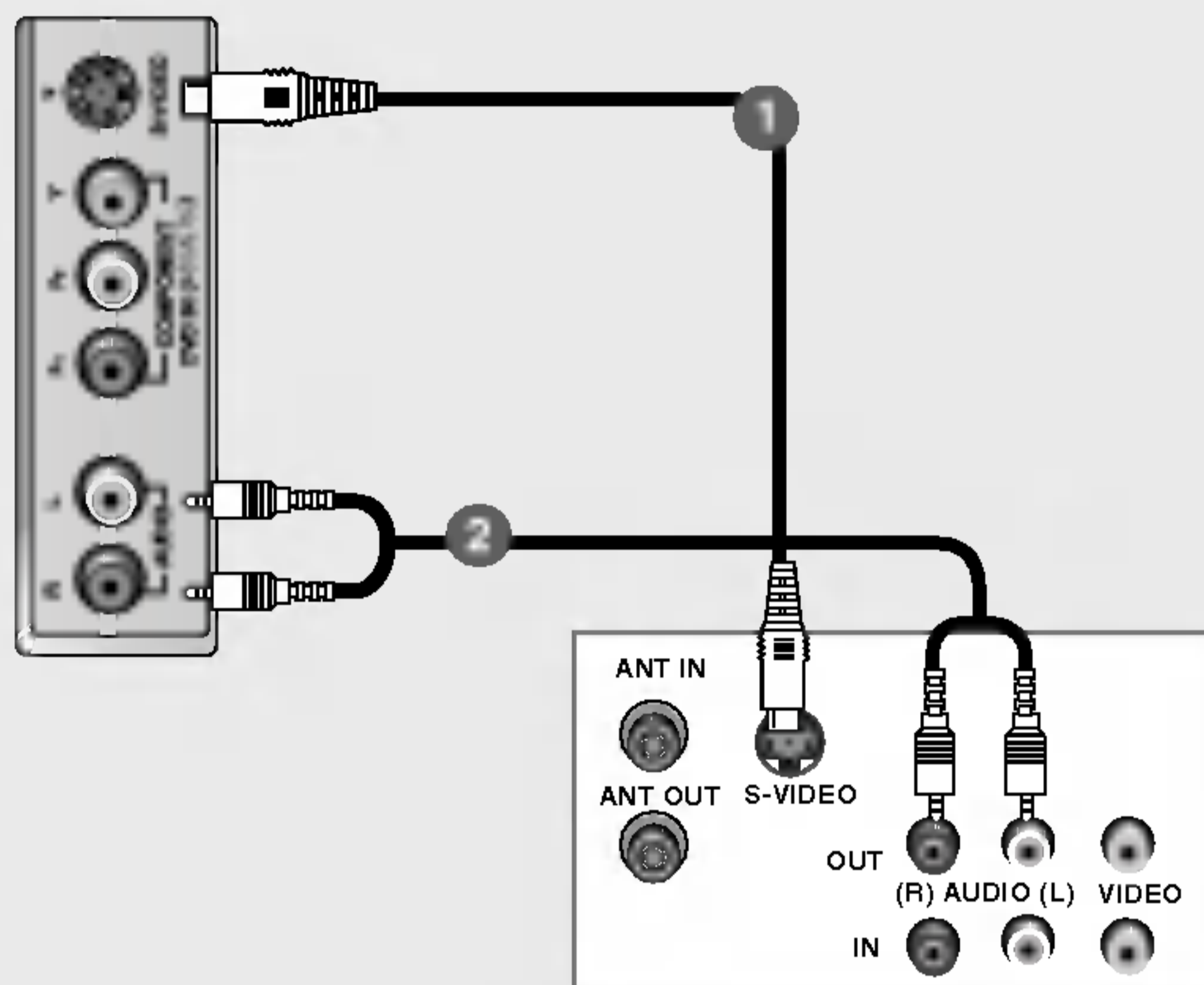
Видеомагнитофон
