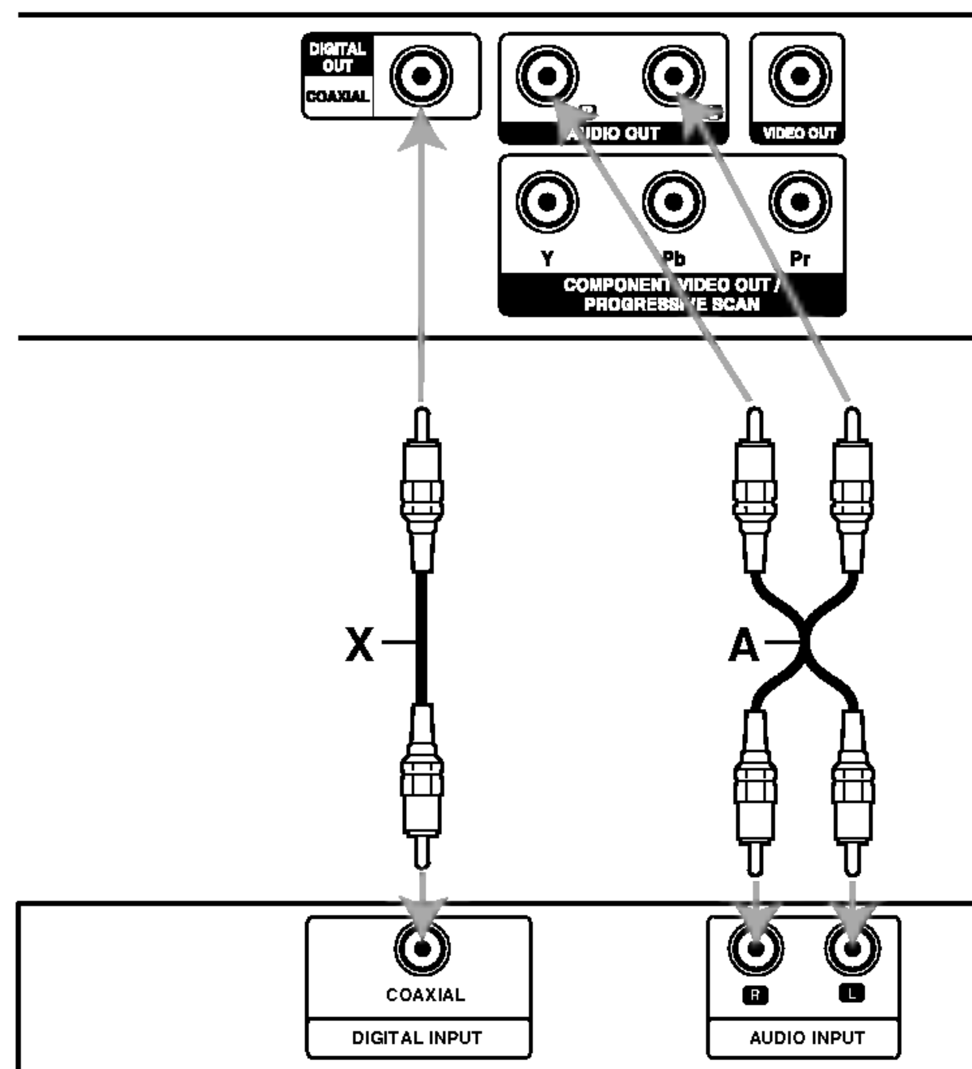
Zesilovač (přijímač)
