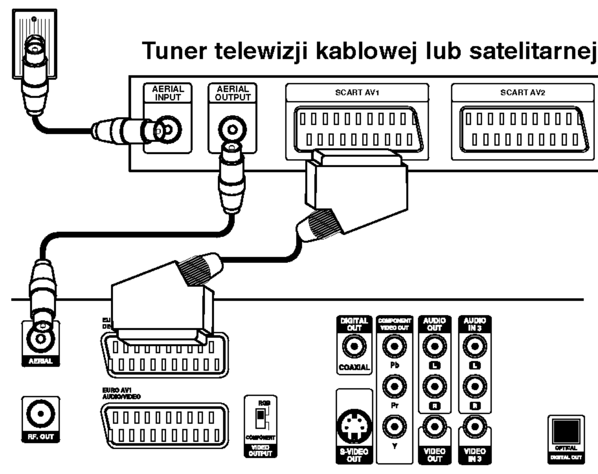
Tył nagrywarki
