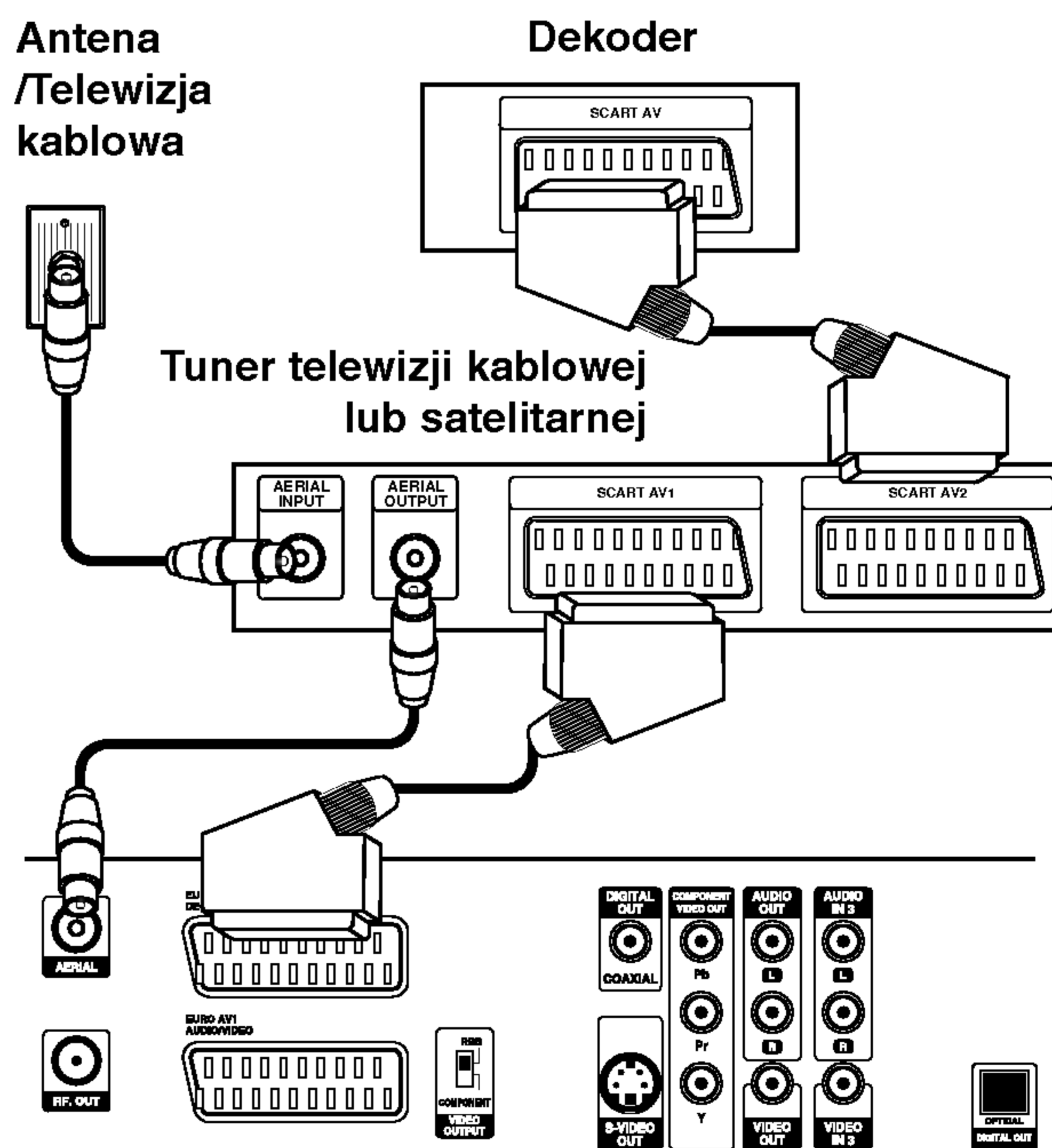
Tył nagrywarki
