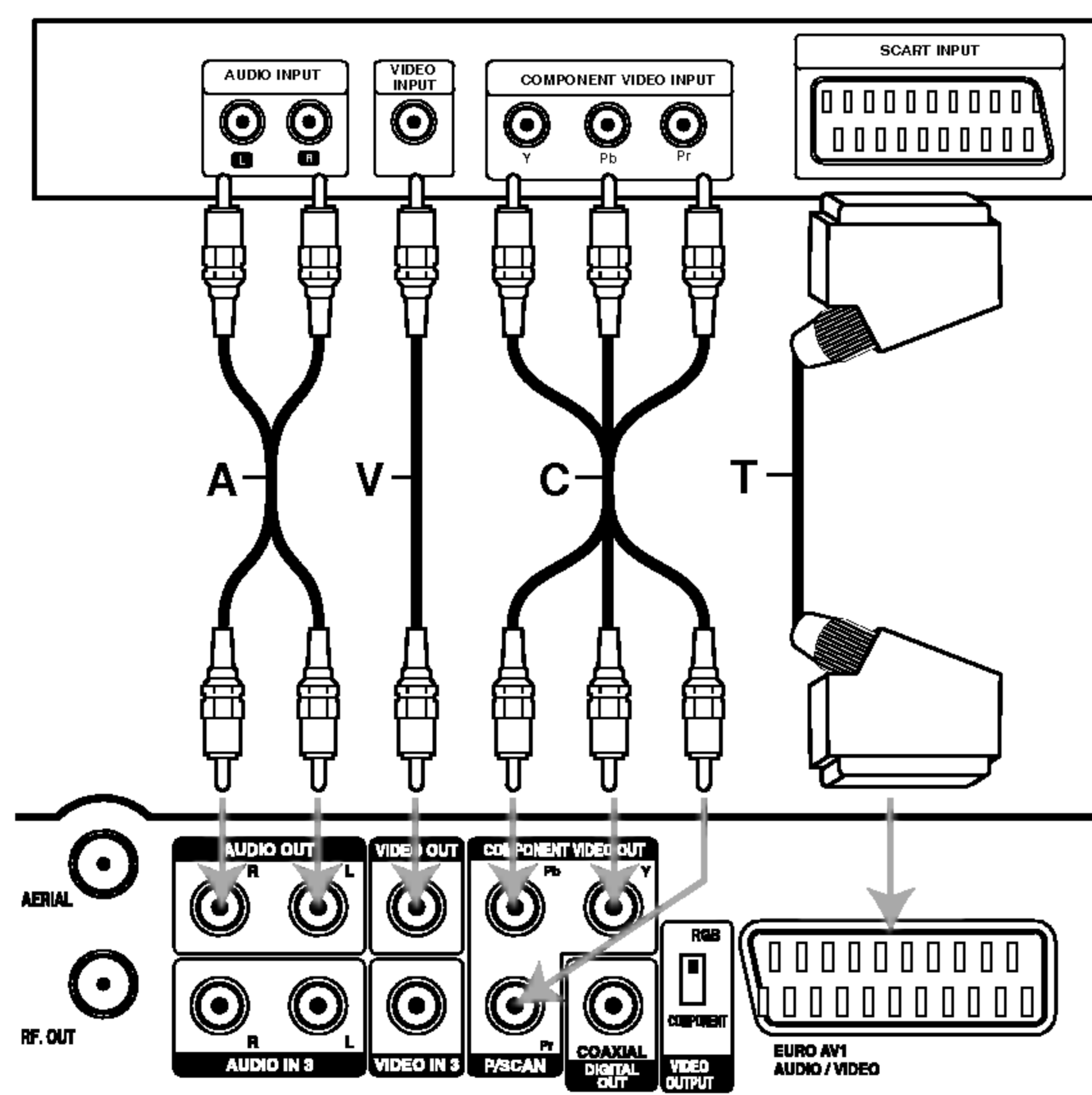
Parte posterior de la grabadora
