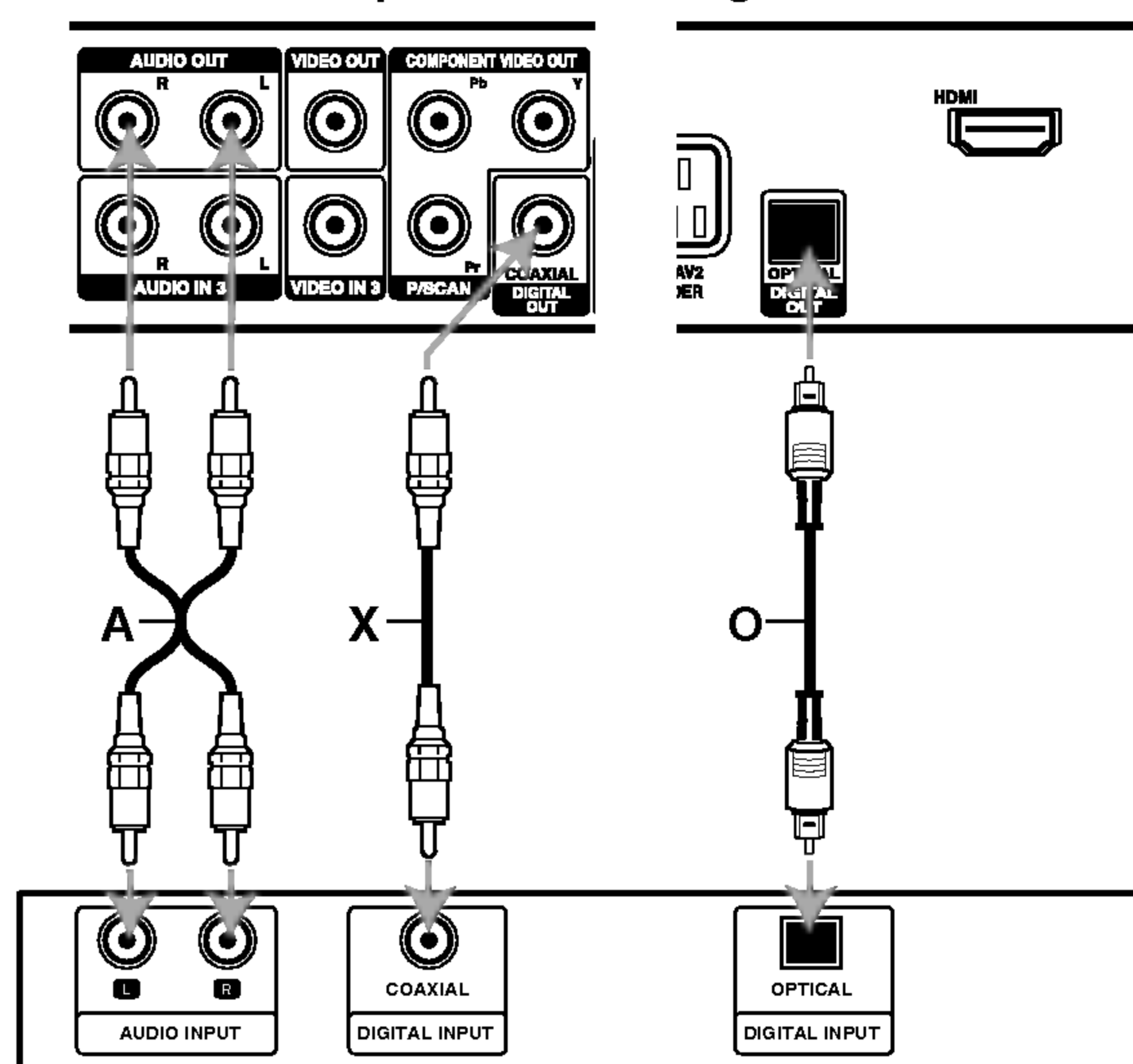
Amplificador (Receptor)
