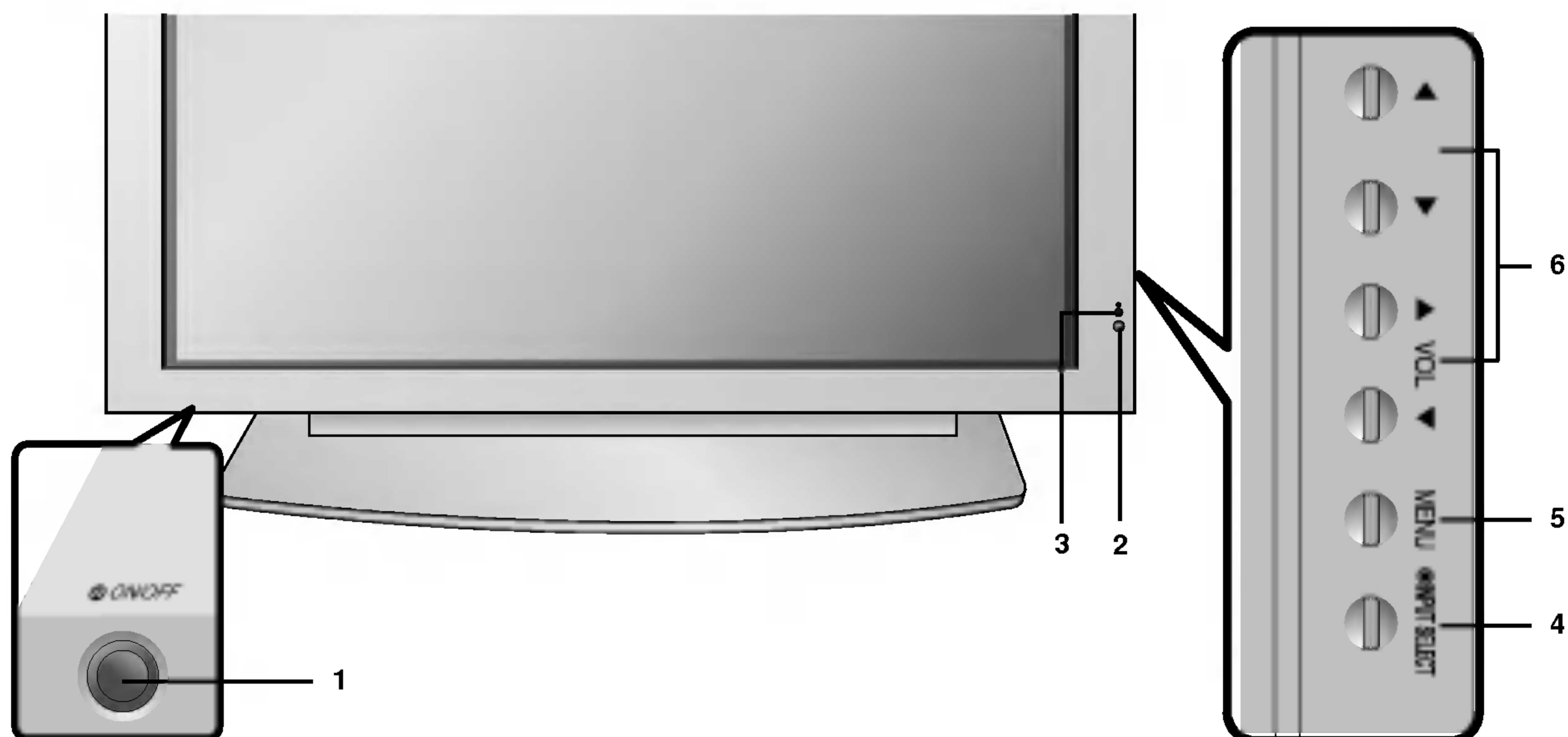
< Panel czołowy >
