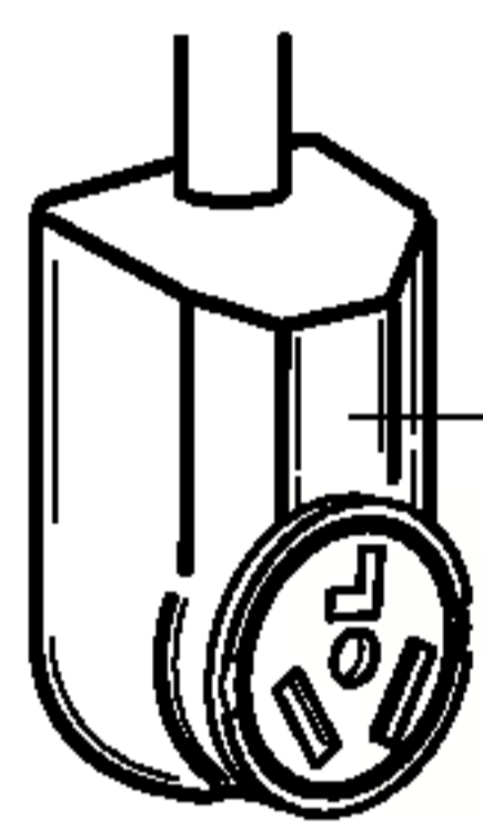
Tomacorriente de 3-alambres (Tipo NEMA 10-30R)
