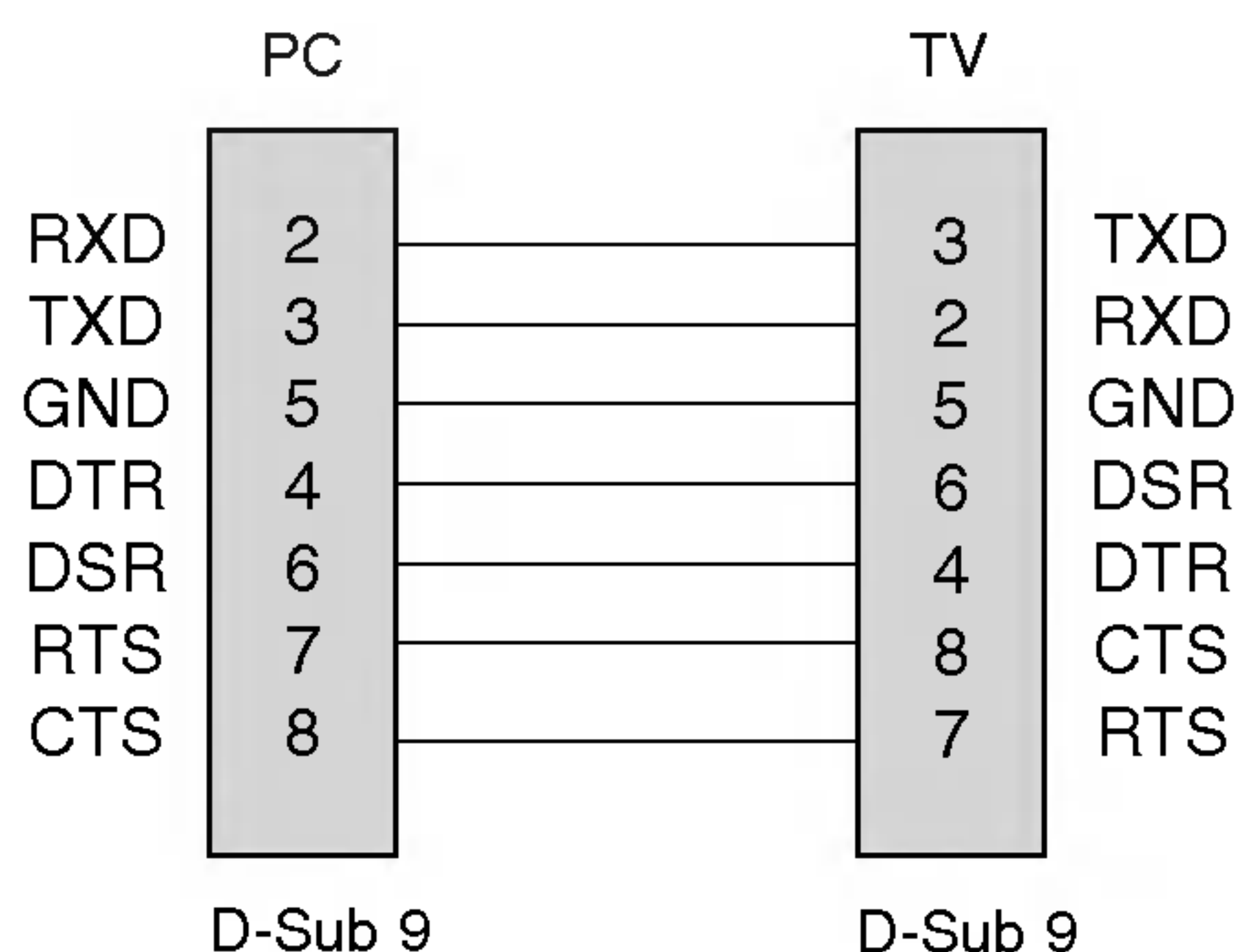
Configurations 7 fils (câble RS-232C standard)
