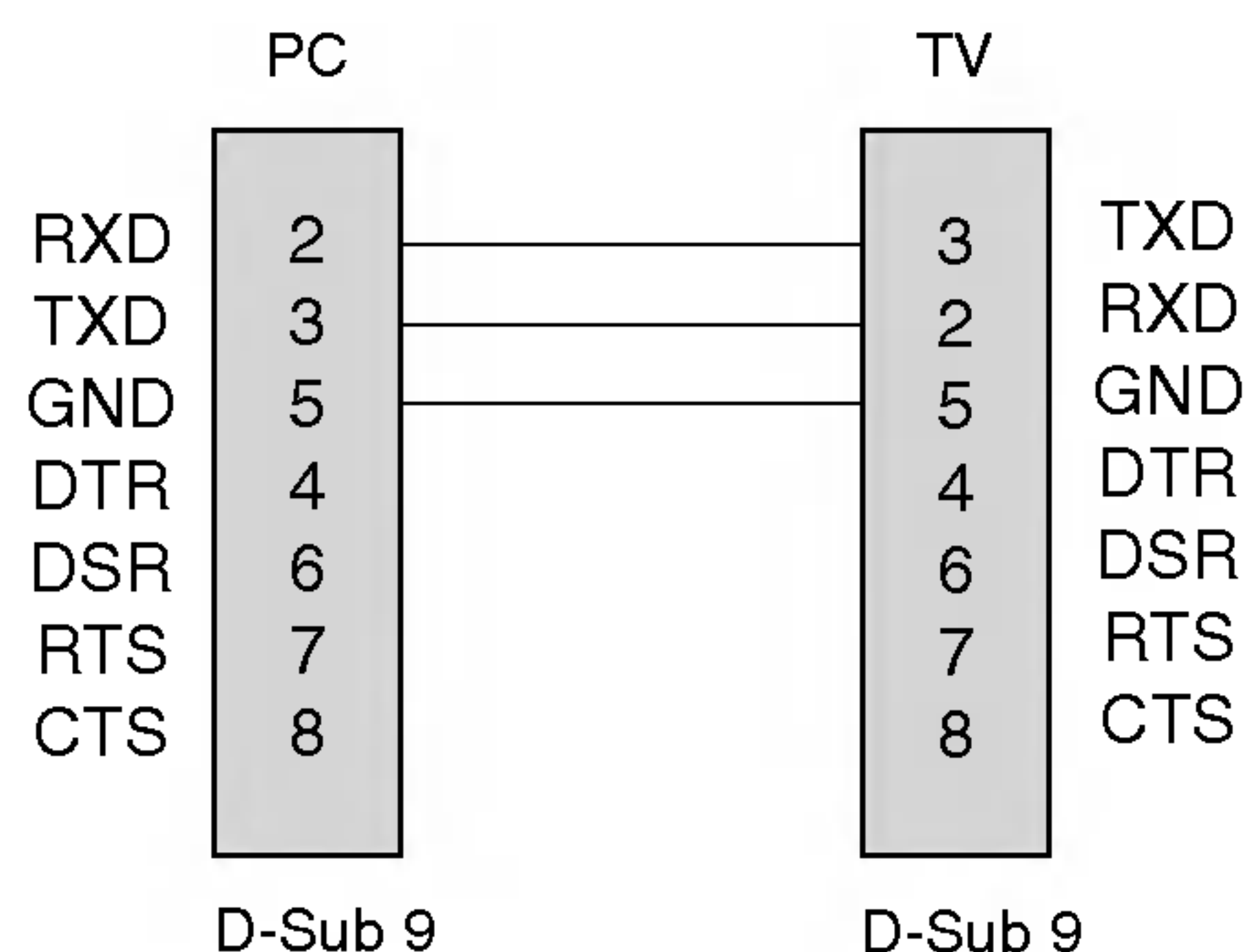
Configurations 3 fils (non standard)
