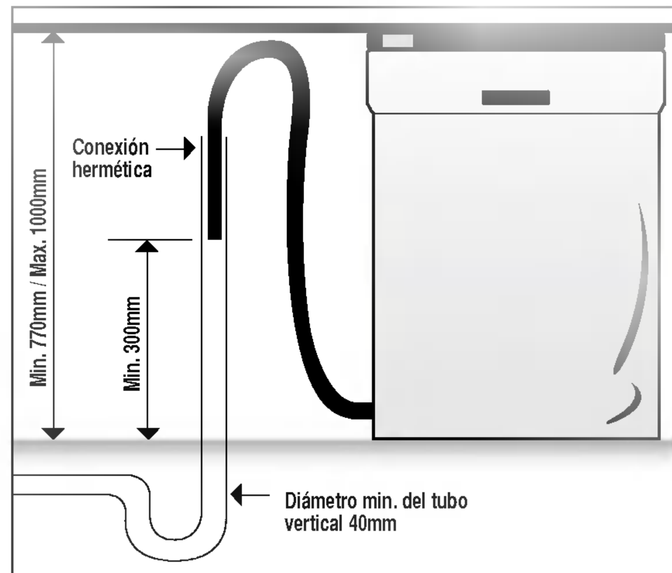
Fig. B: Conexión de desagüe - tubo vertical.
