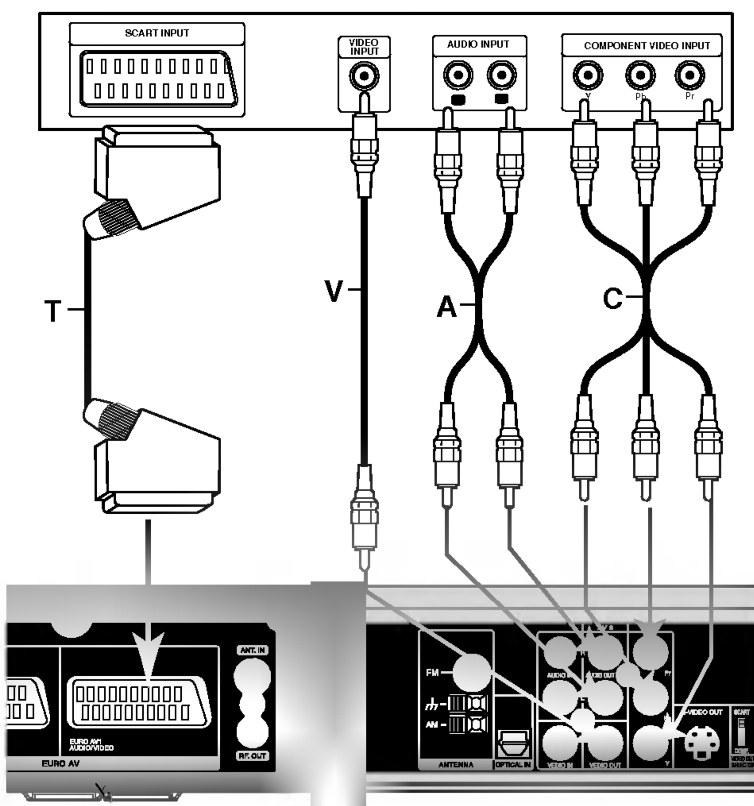
Zadnja strana DVD rekorder prijemnika
