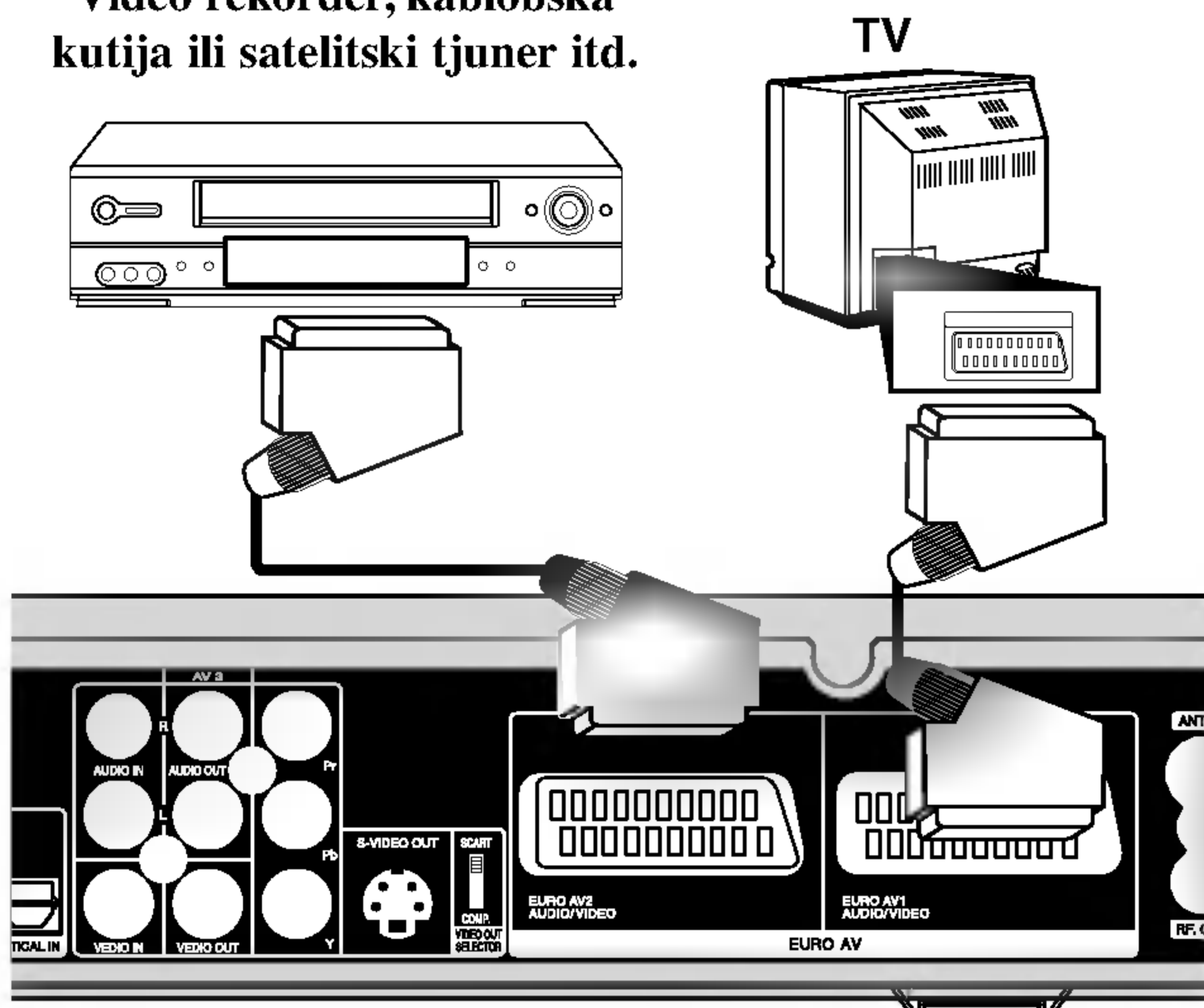
Zadnja strana DVD rekorder prijemnika
