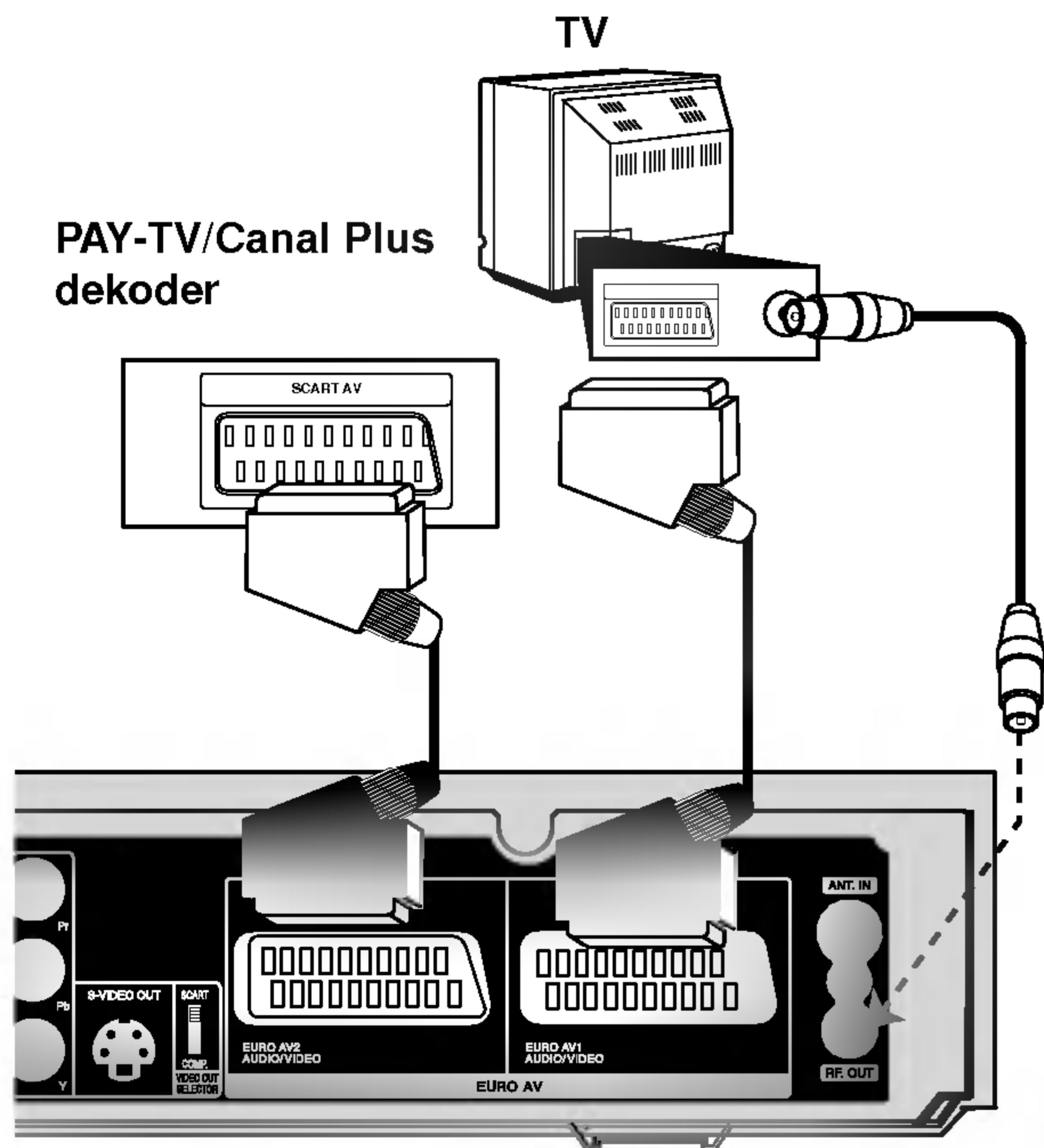
Bagsiden af DVD optageren/modtageren
