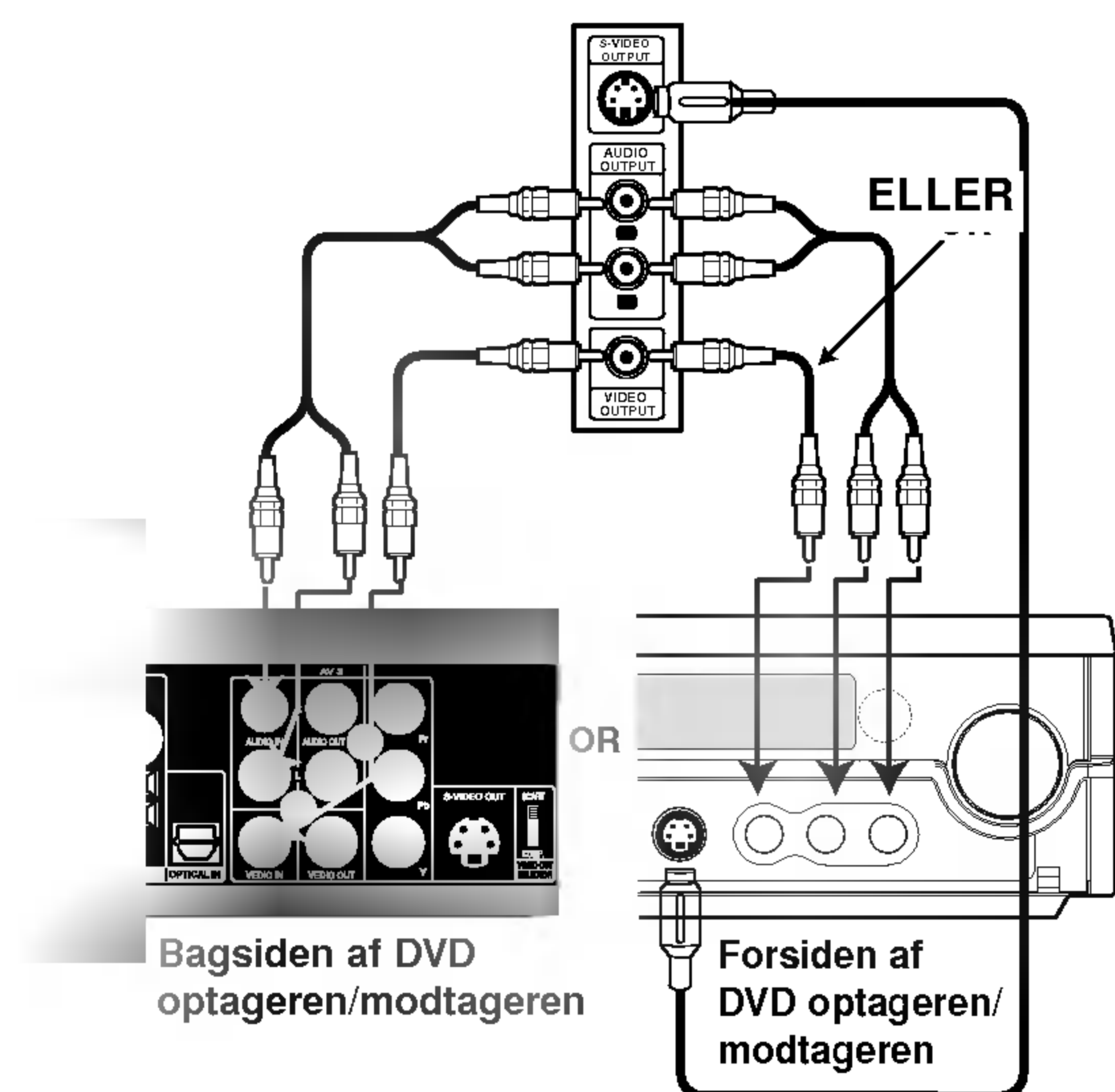
Jack-panel på den ekstra komponent (VCR, videokamera osv.).
