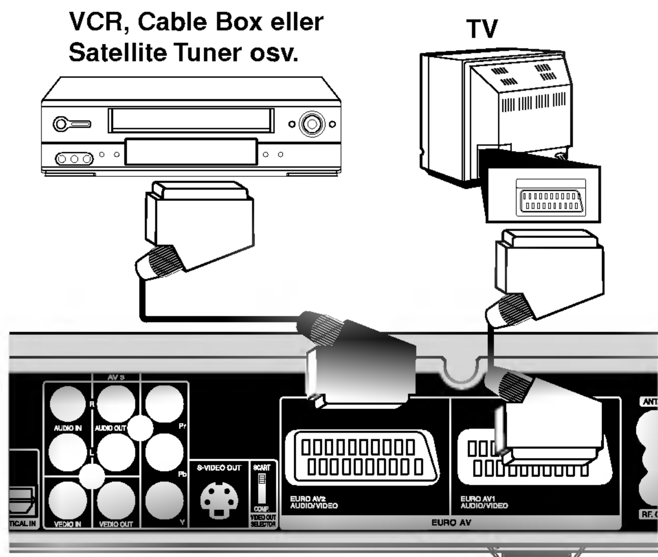
Bagsiden af DVD optageren/modtageren
