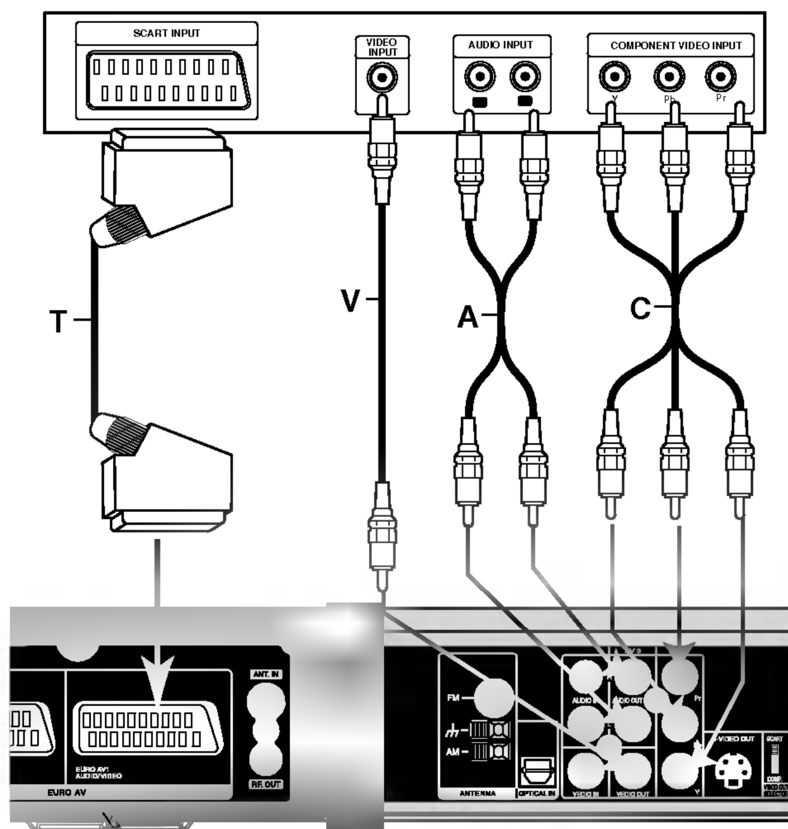
Bagsiden af DVD optageren/modtageren
