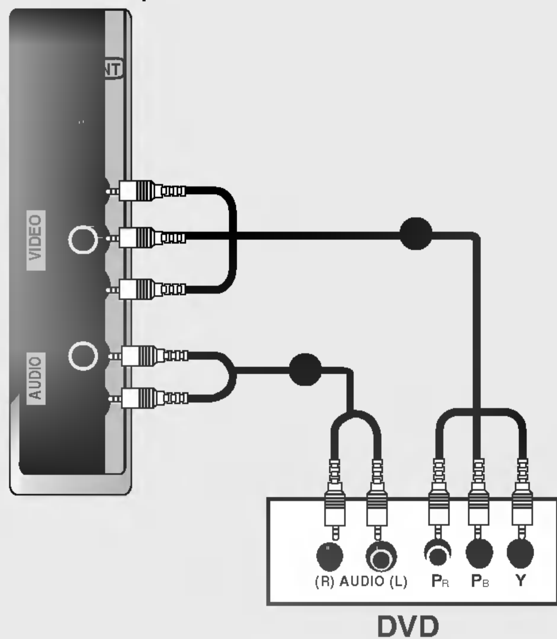
Страничен панел на телевизора
