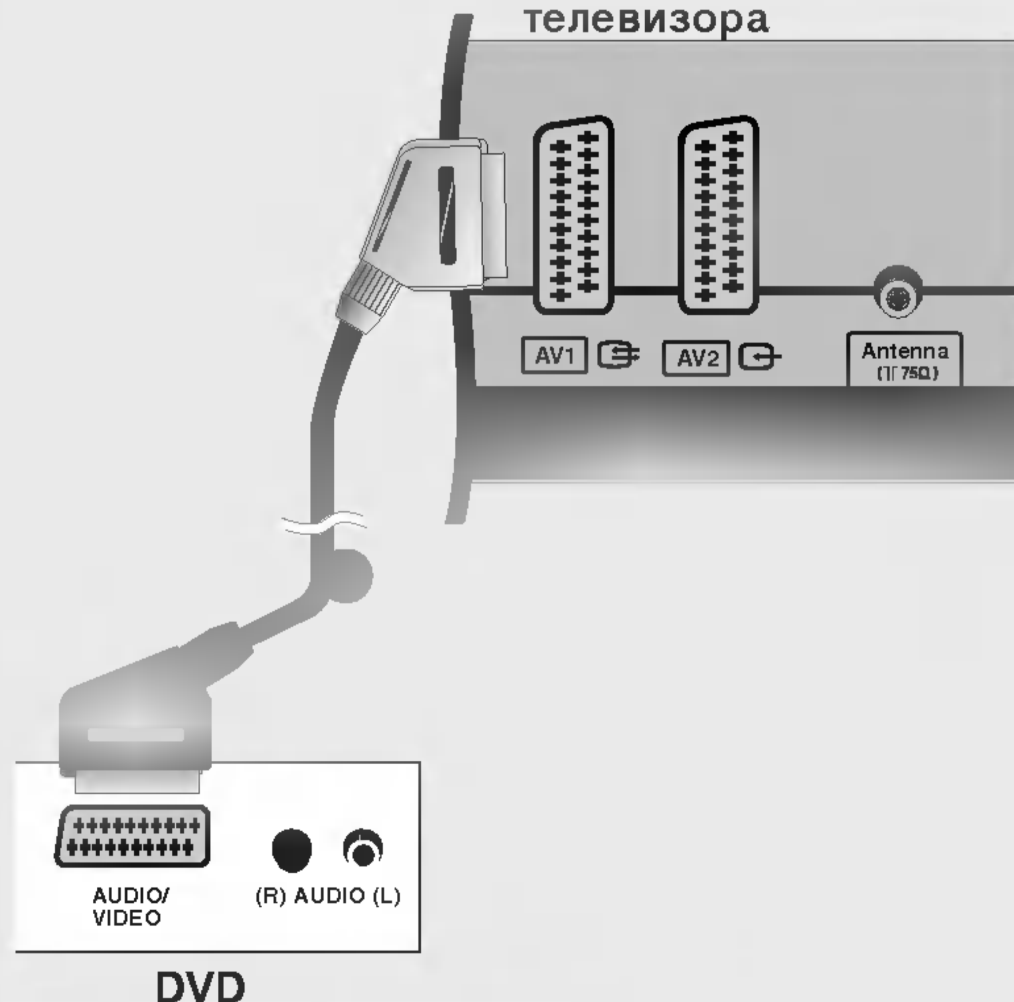
Заден панел на телевизора
