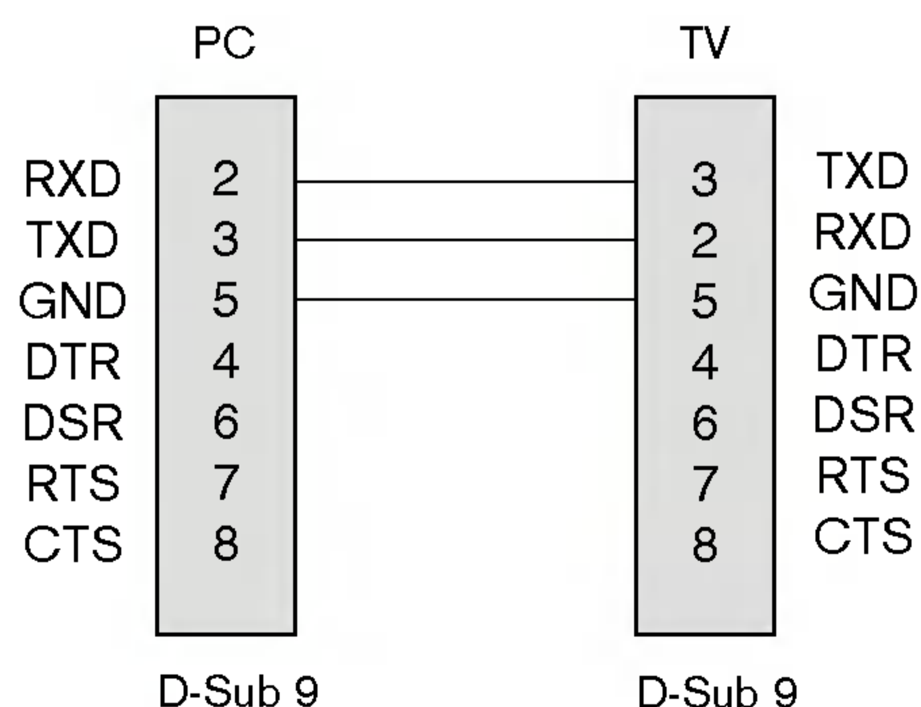
Konfiguracje 3-żyłowe (niestandardowe)
