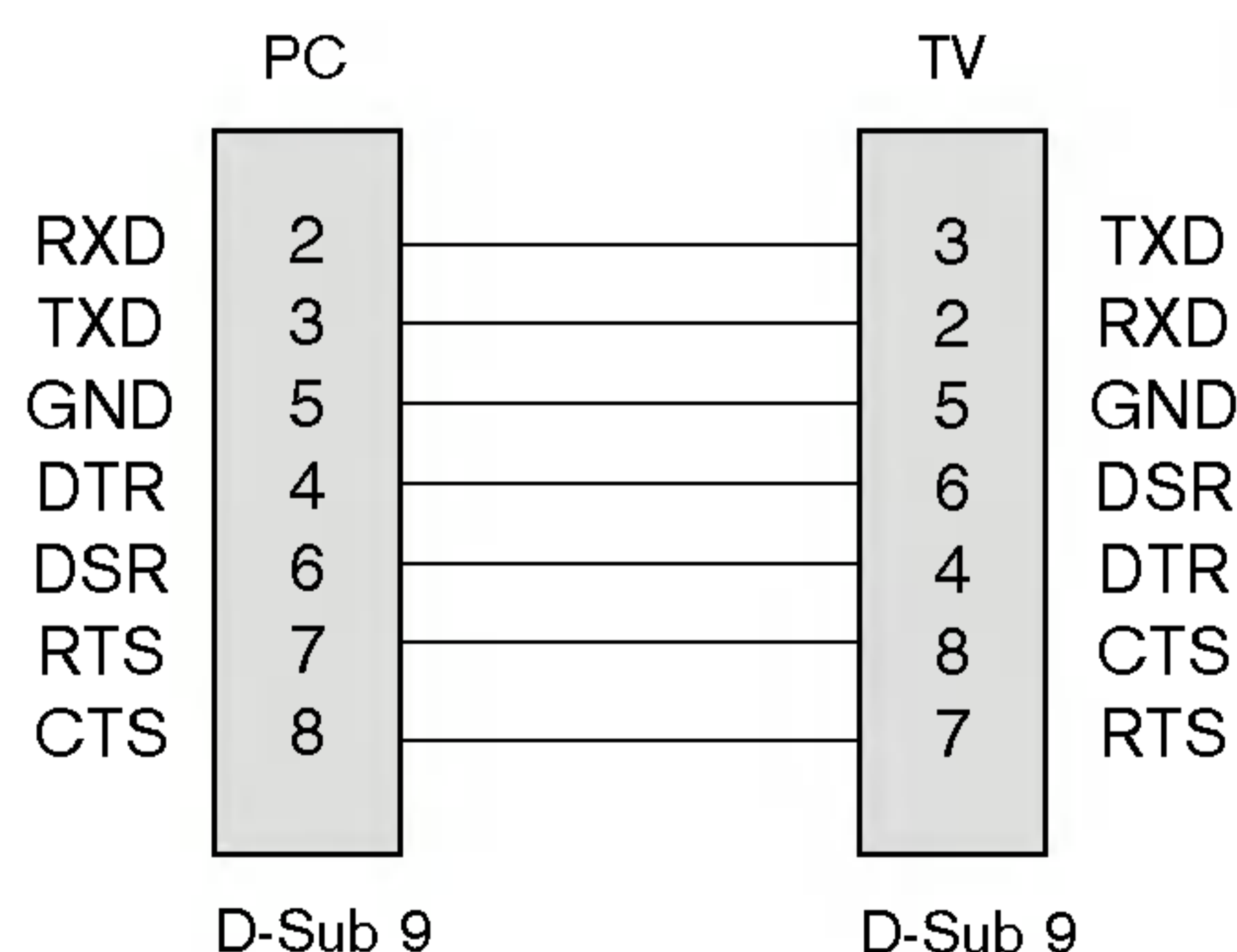
Konfiguracje 7-żyłowe (standardowy kabel RS-232C)
