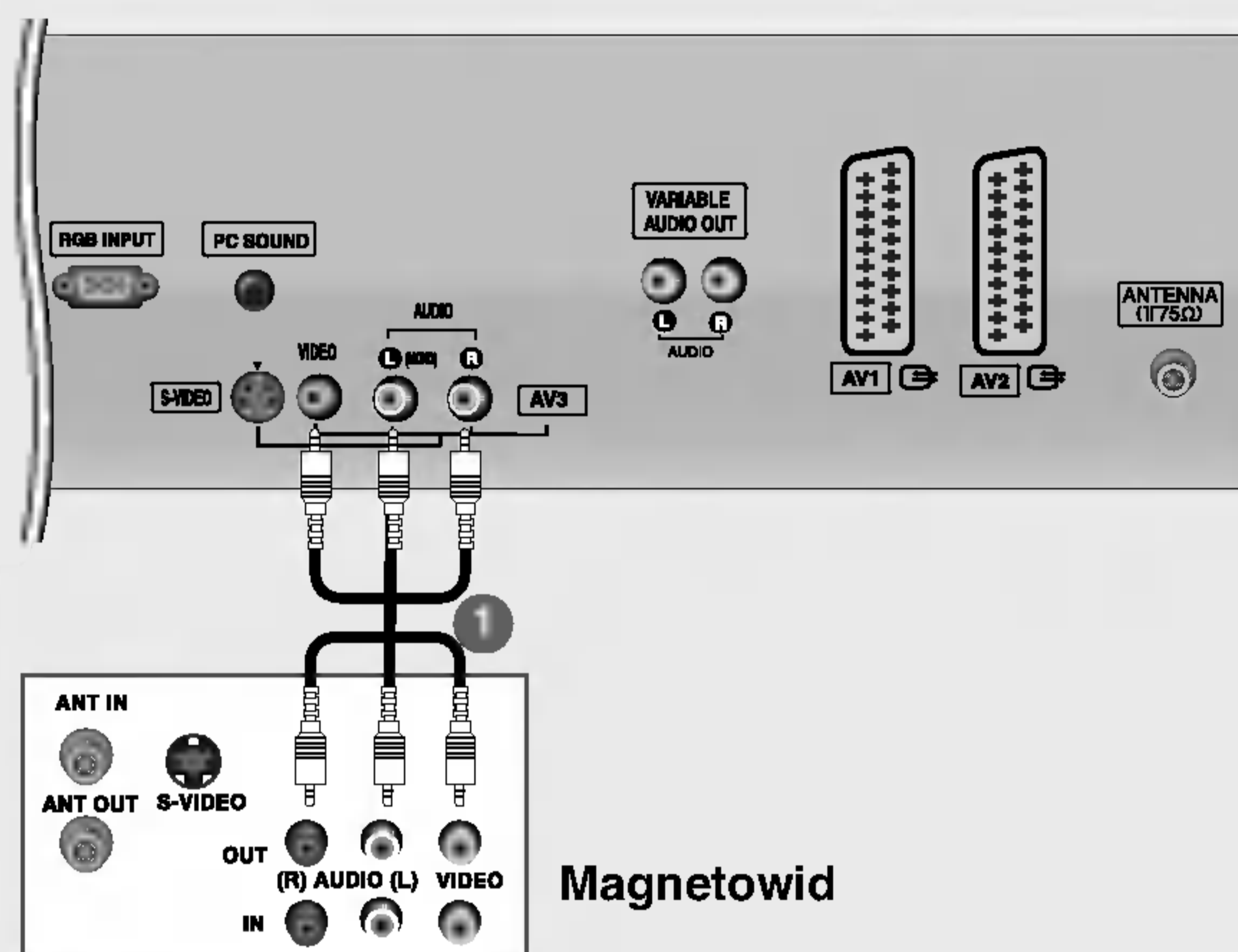
Panel tylny telewizora
