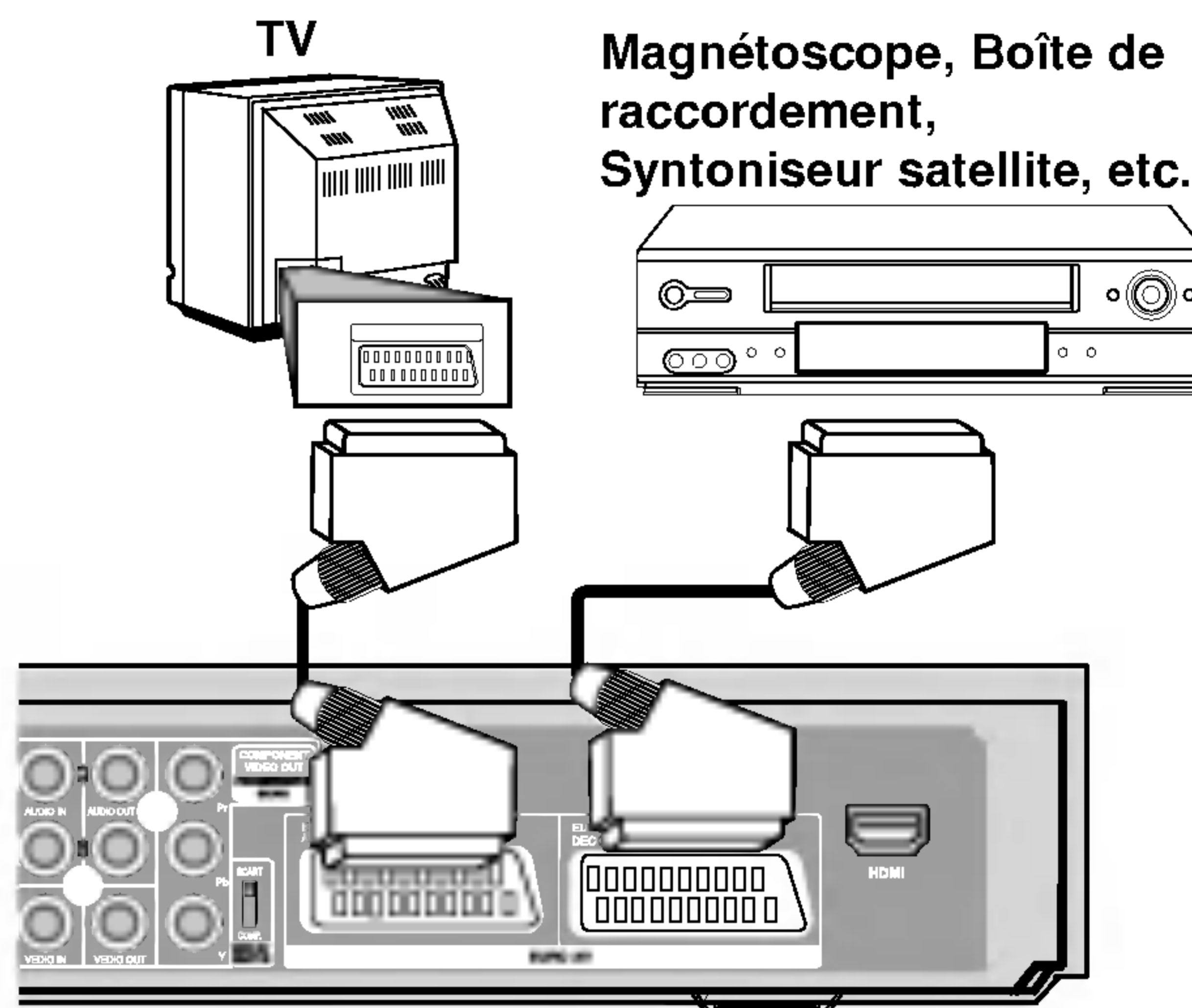
L'arrière du Récepteur Enregistreur HDD/DVD
