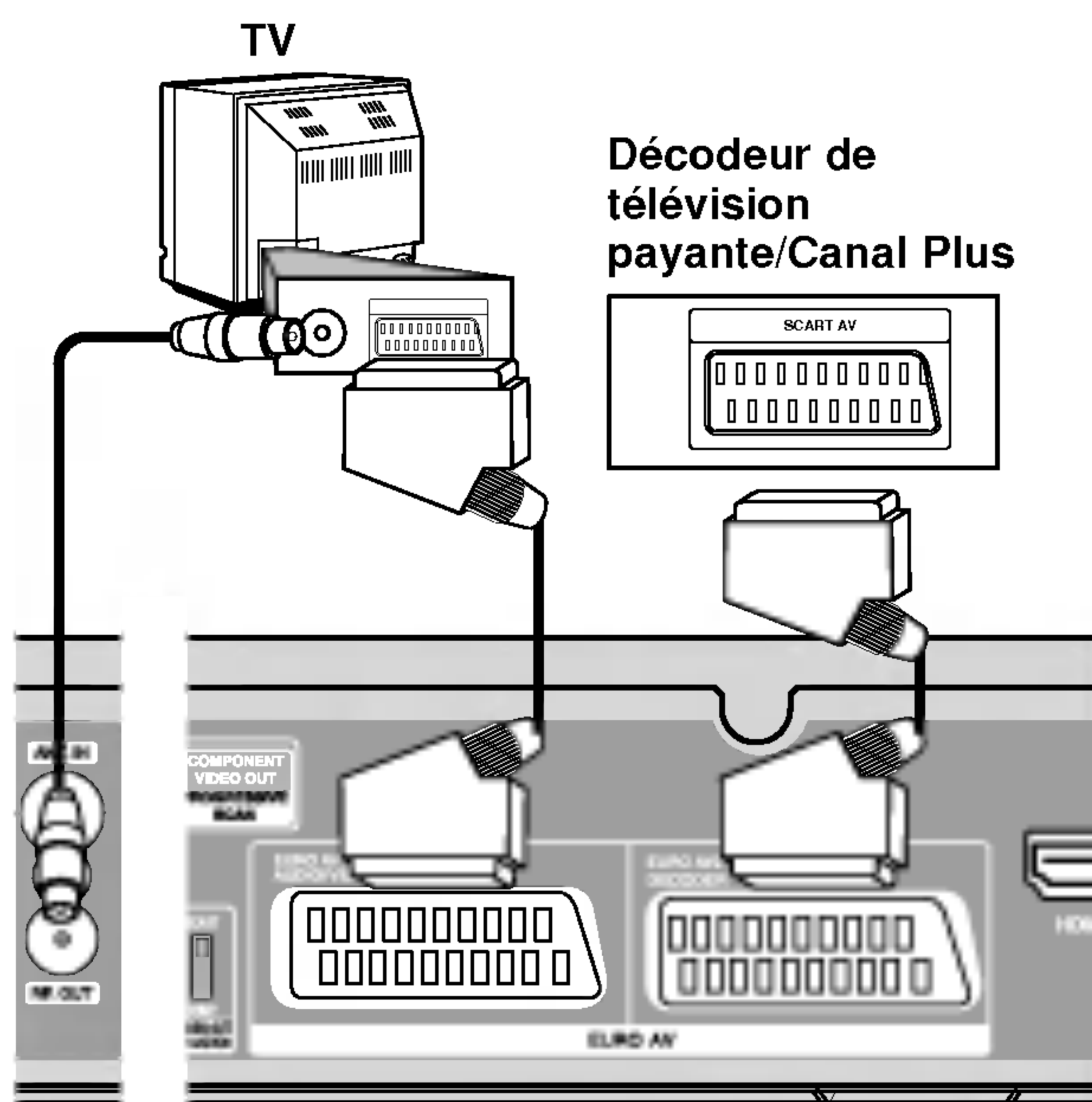
L'arrière du Récepteur Enregistreur HDD/DVD
