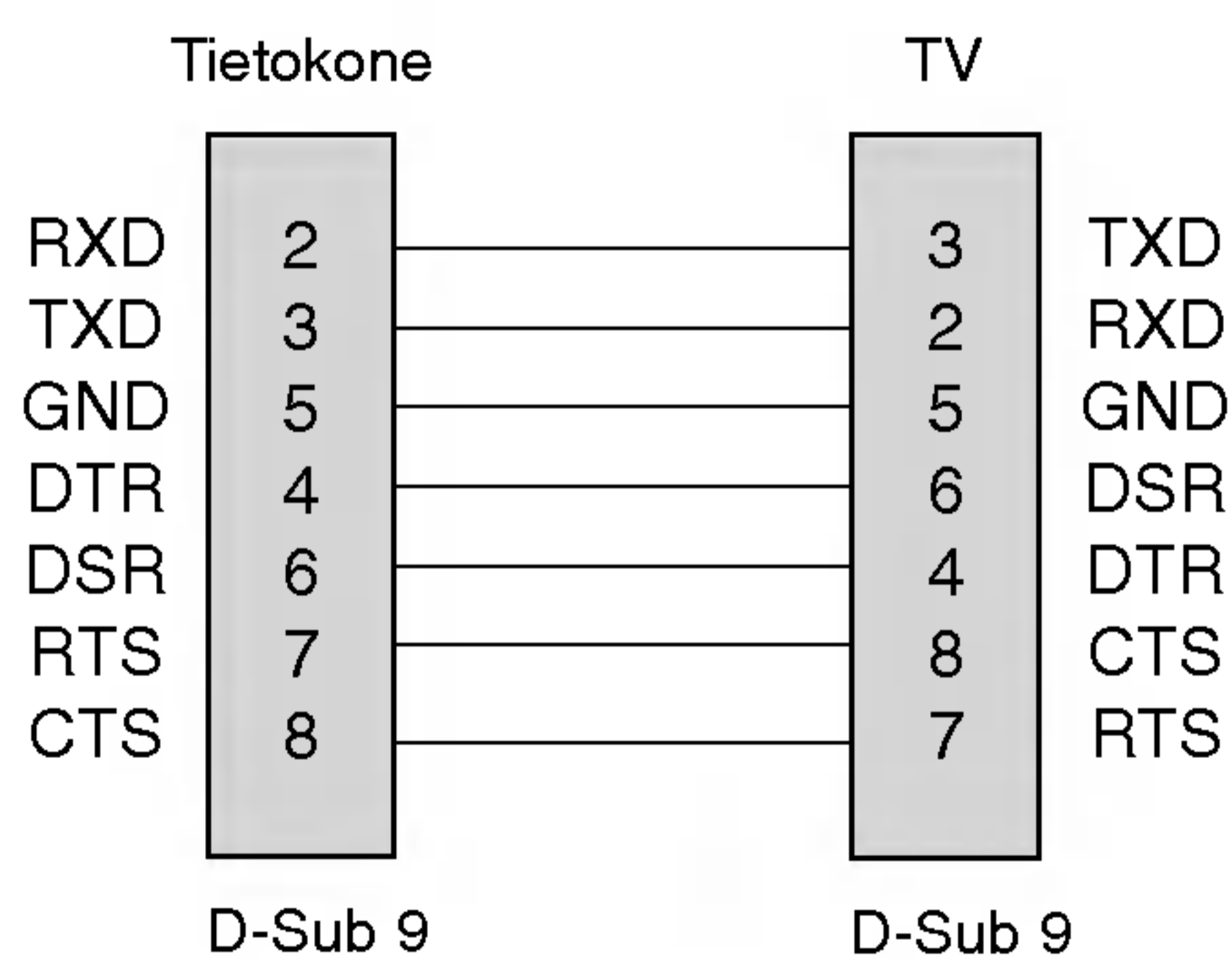
7-johtiminen kytkentä (RS-232C -kaapelin vakiokytkentä)
