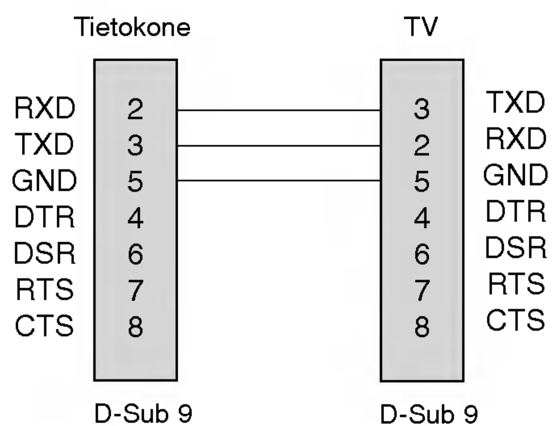
3-johtiminen kytkentä (ei vakiokytkentä)
