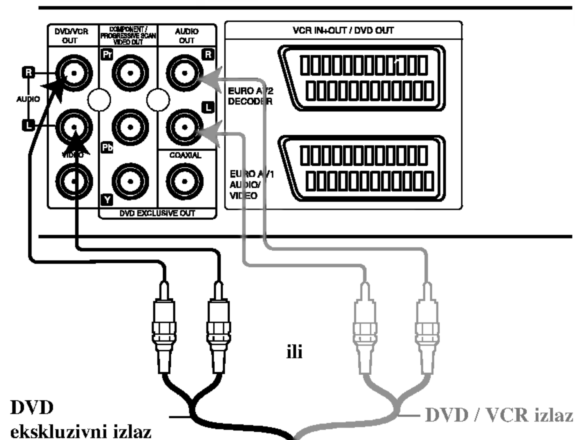
Stražnji dio ovog uređaja
