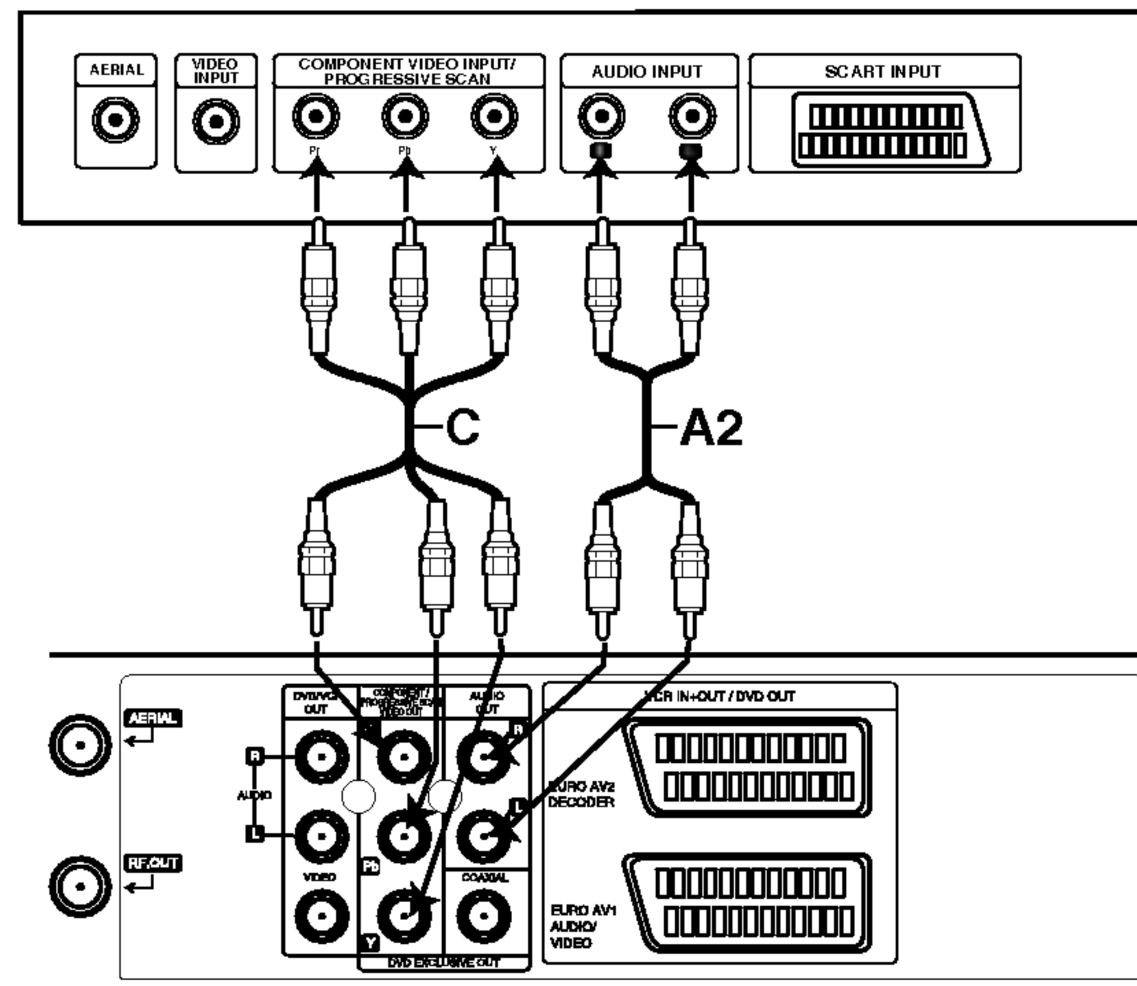
Stražnji dio ovog uređaja (Osnovni priključak)
