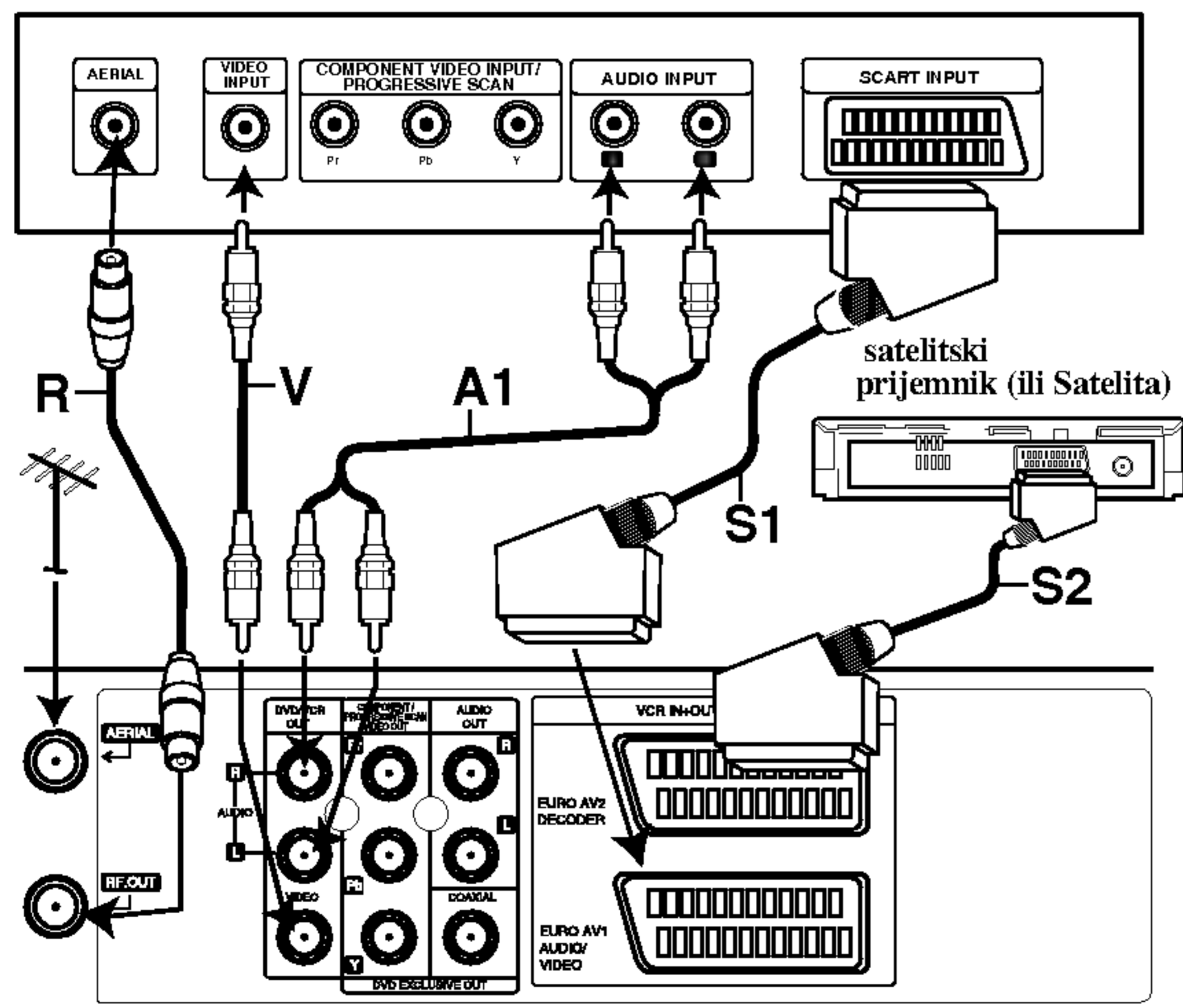
Stražnji dio ovog uređaja (Osnovni priključak)
