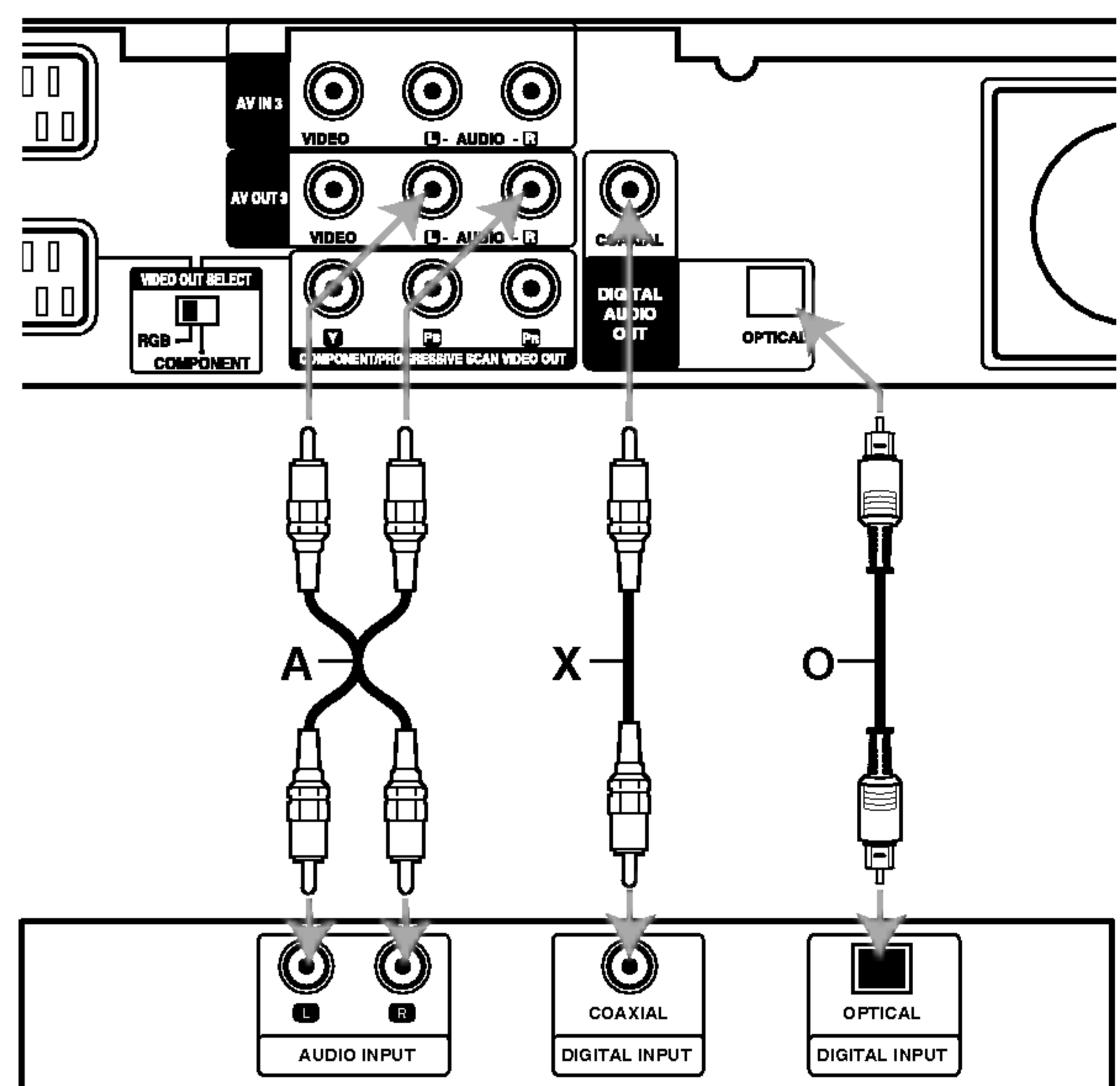
Verstärker (Receiver)
