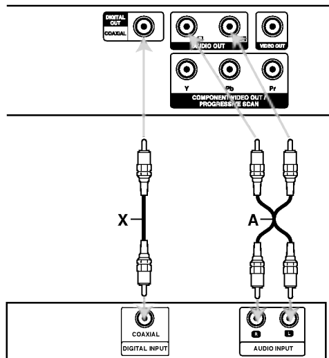
Усилвател (приемник)
