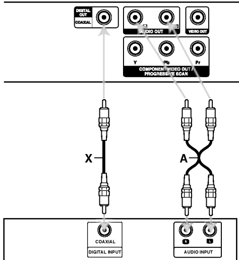
Pojačivač (prijemnik)
