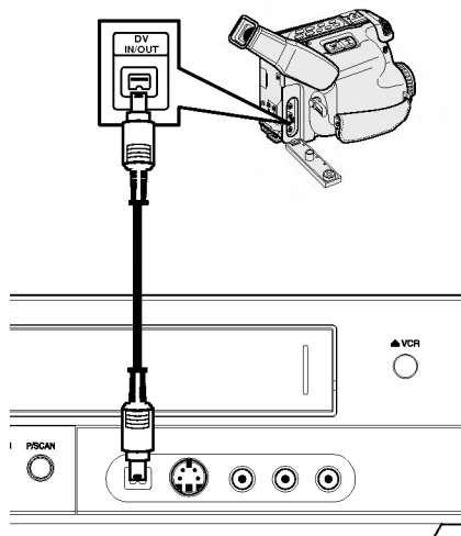
Предна страна на рекордера
