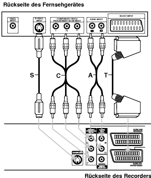
Rückseite des Recorders
