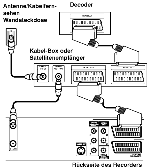
Rückseite des Recorders
