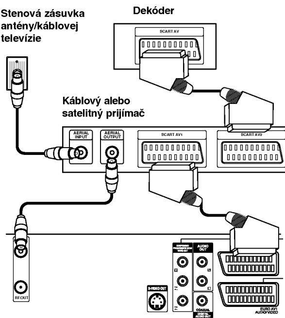
Zadný panel rekordéra
