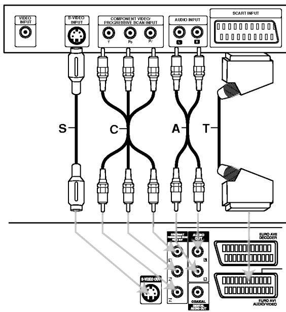
Zadný panel rekordéra
