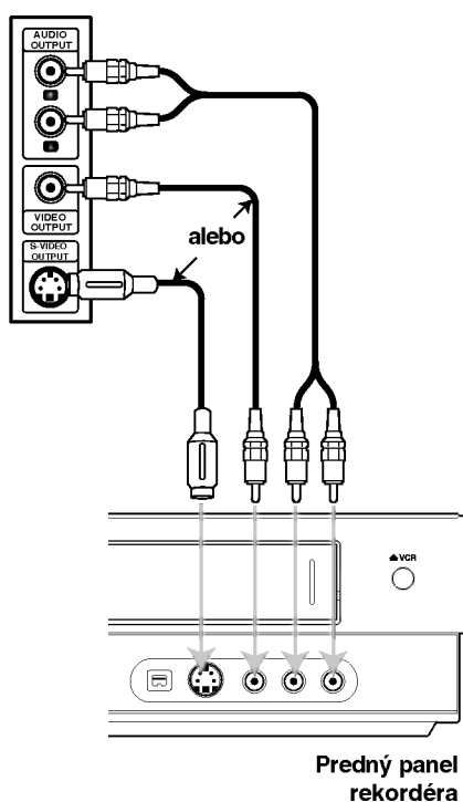
Panel koncoviek prídavného zariadenia (video rekordér, kamera atď.)
