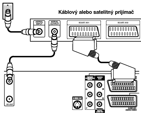
Zadný panel rekordéra
