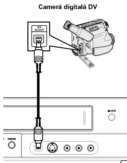
Partea din față a recorderului
