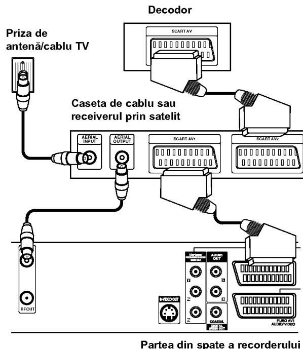
Partea din spate a recorderului
