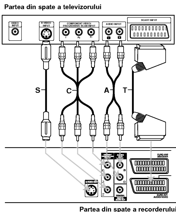
Partea din spate a recorderului
