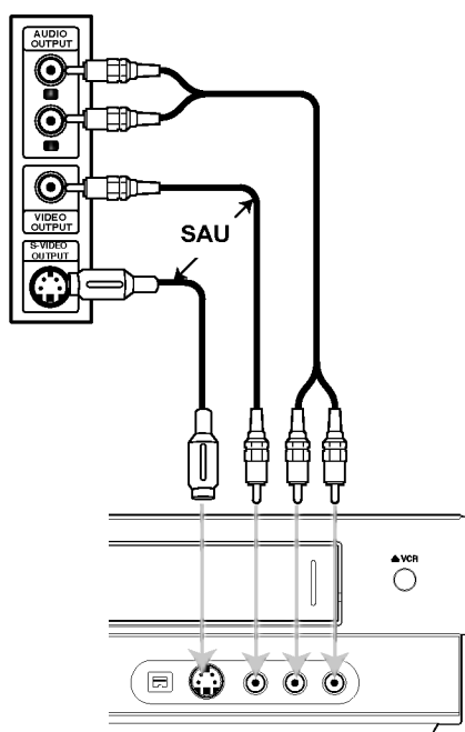
Partea din față a recorderului
