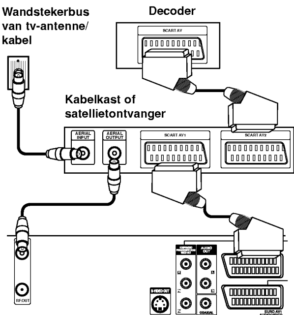
Achterkant van recorder
