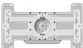
Wandhalterung, neigbar
