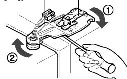
Övre gångjärn
