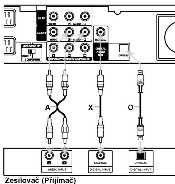
Zadní část rekordéru
