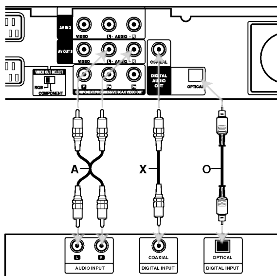
Zosilňovač (Prijímač)
