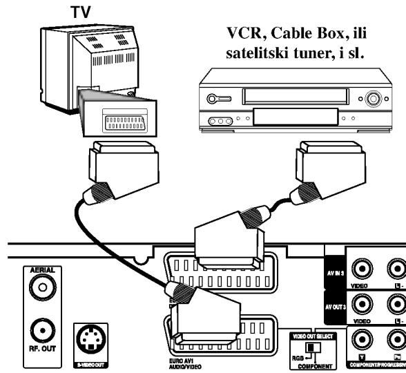
Zadnja strana rekordera
