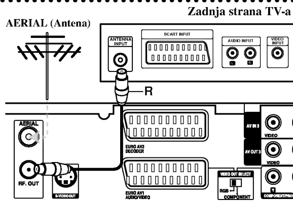
Zadnja strana rekordera
