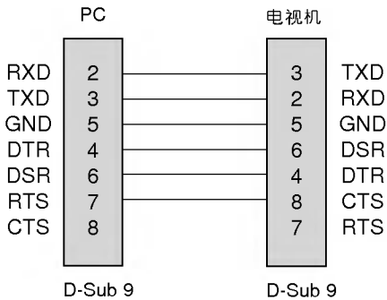
7股线的配置 (标准 RS-232C 连接线)
