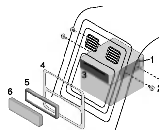
Panel przedni
