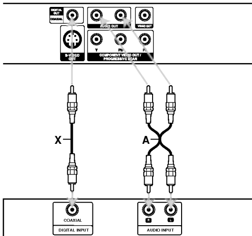
Amplificador (Receptor)
