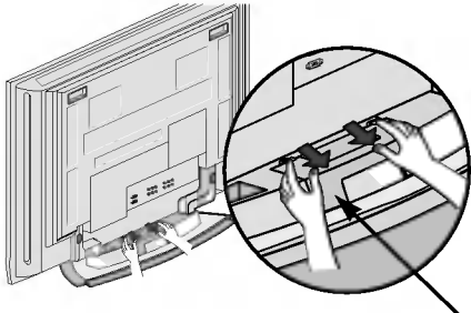
ماسك الكابلات
