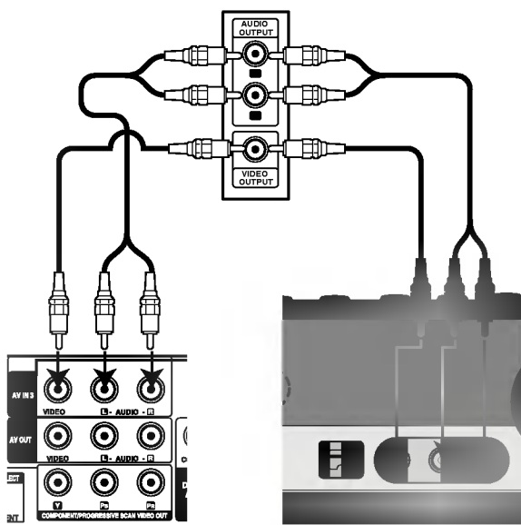
Zadná strana HDD/DVD rekordéra
