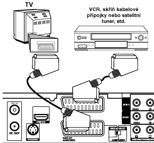
Zadní část HDD/DVD rekordéru s přijímačem
