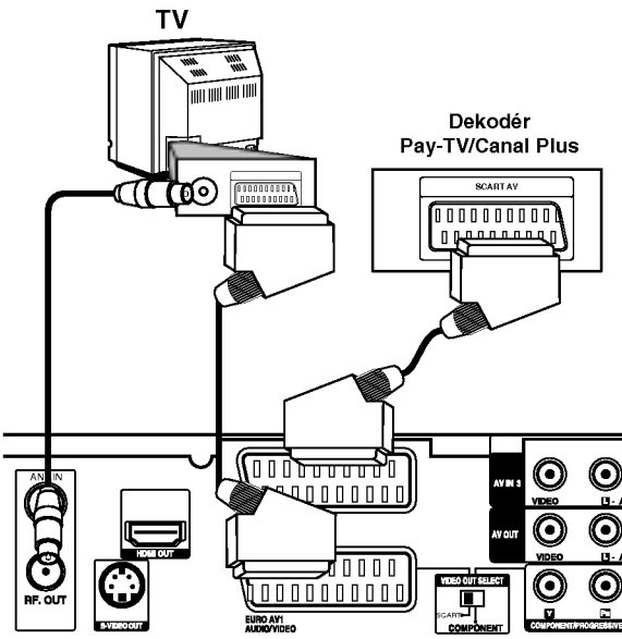
Zadní část HDD/DVD rekordéru s přijímačem
