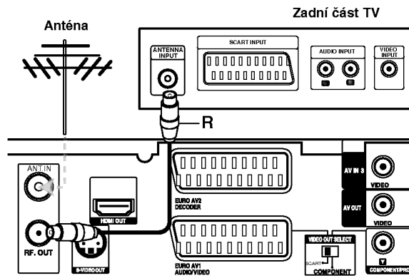
Zadní část HDD/DVD rekordéru s přijímačem
