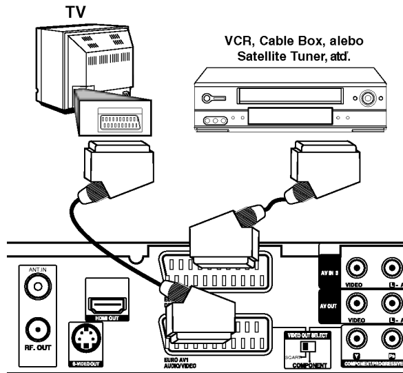
Zadná strana HDD/DVD rekordéra
