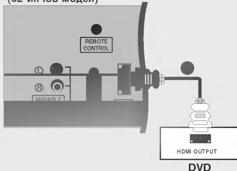
Заден панел на телевизора (32-инчов модел)
