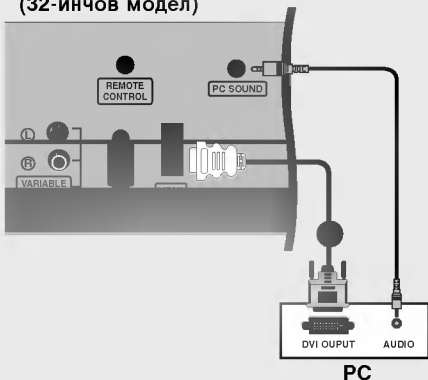
Заден панел на телевизора (32-инчов модел)
