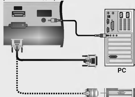
Заден панел на телевизора (26-инчов модел)
