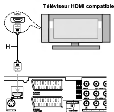
L'arrière du Récepteur Enregistreur HDD/DVD
