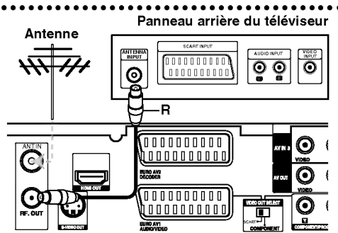
L'arrière du Récepteur Enregistreur HDD/DVD
