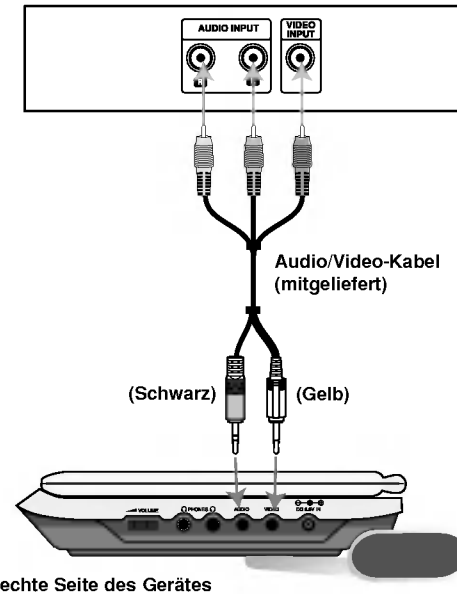
Rückseite des Fernsehgerätes
