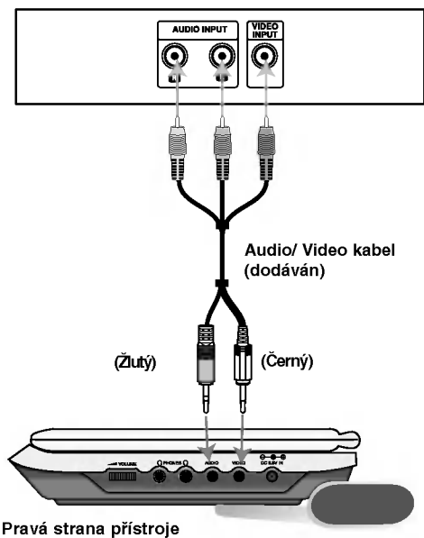
Zadní panel televizoru
