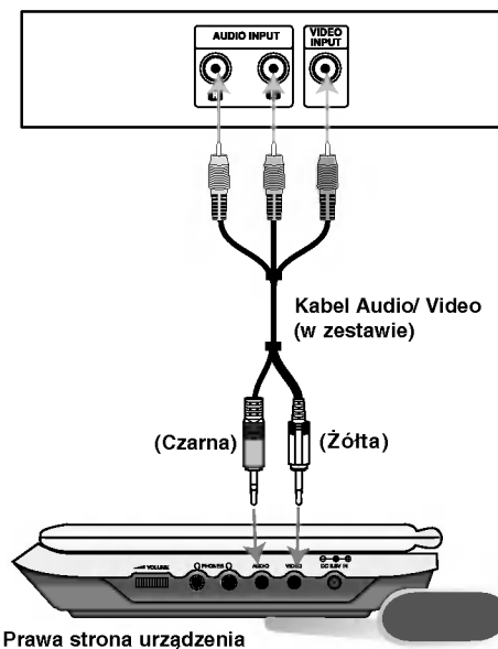
Tył telewizora
