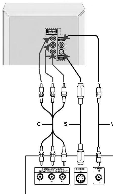
Parte posterior TV
