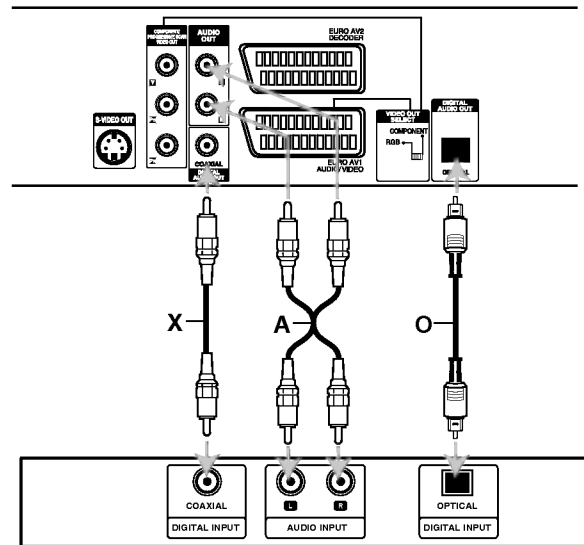
Vahvistin (vastaanotin)
