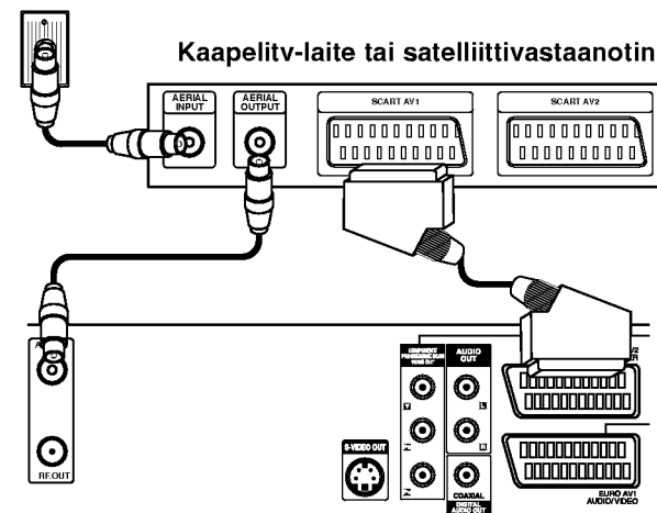
Tallennin takaa
