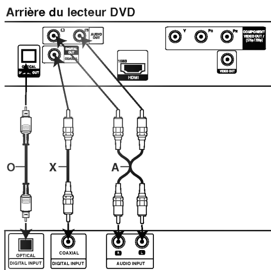
Amplificateur (Récepteur)
