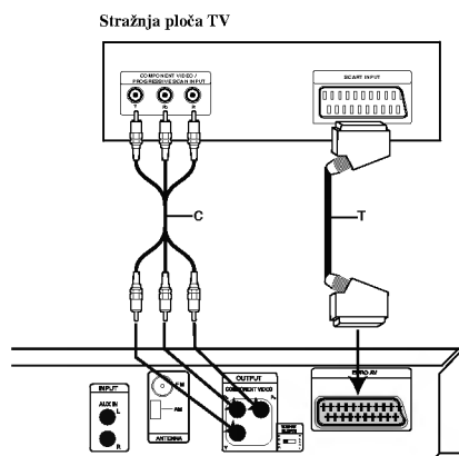
Stražnji dio DVD/CD prijemnika
