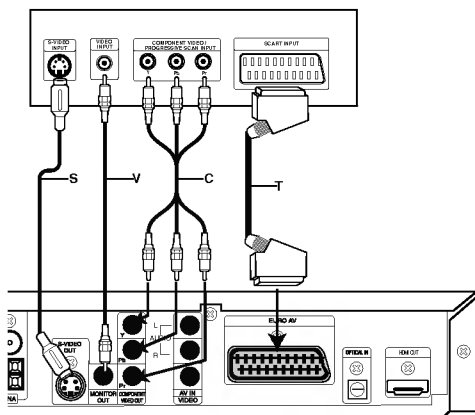
Rückseite des DVD/CD-Receiver
