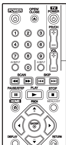
Кнопки управления телевизором
