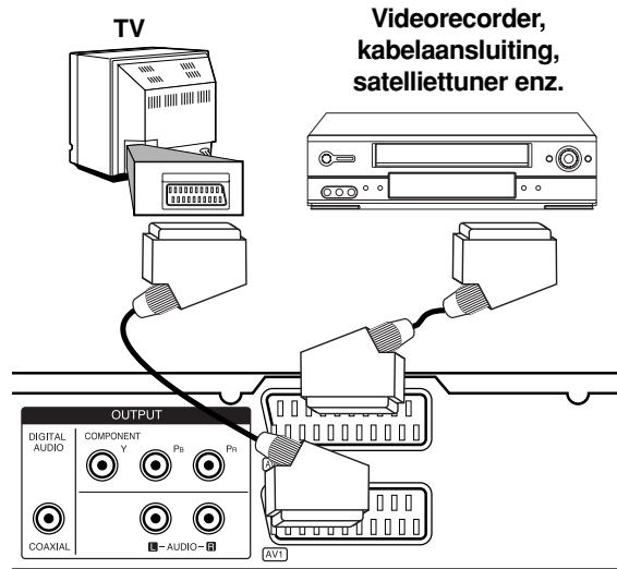
Achterzijde van de recorder
