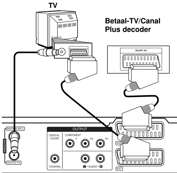
Achterzijde van de recorder
